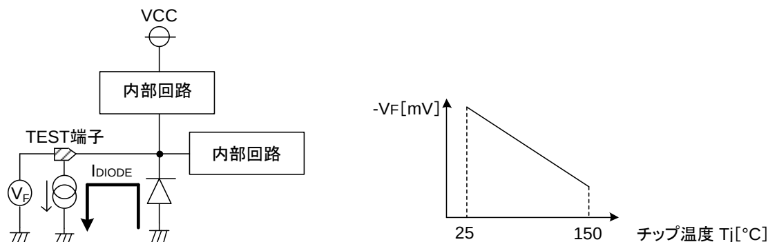
Figure 3. チップ温度測定の様式図
