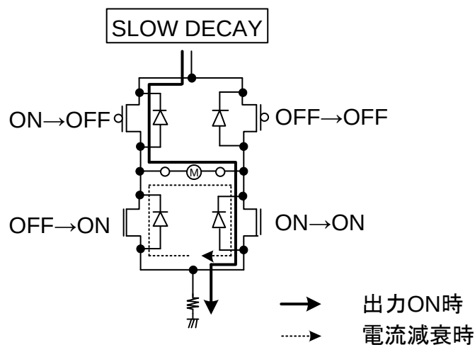
Figure 2. 電流減衰時の回生電流経路
