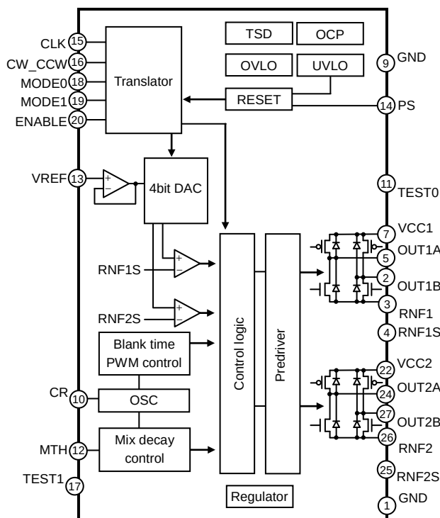
Figure.3 BD63510AEFV ブロック図
