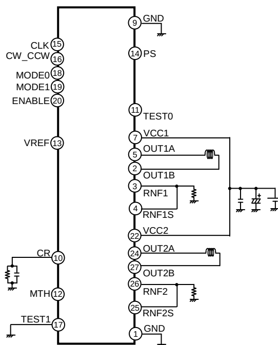
Figure.1 BD63510AEFV アプリケーション回路図
