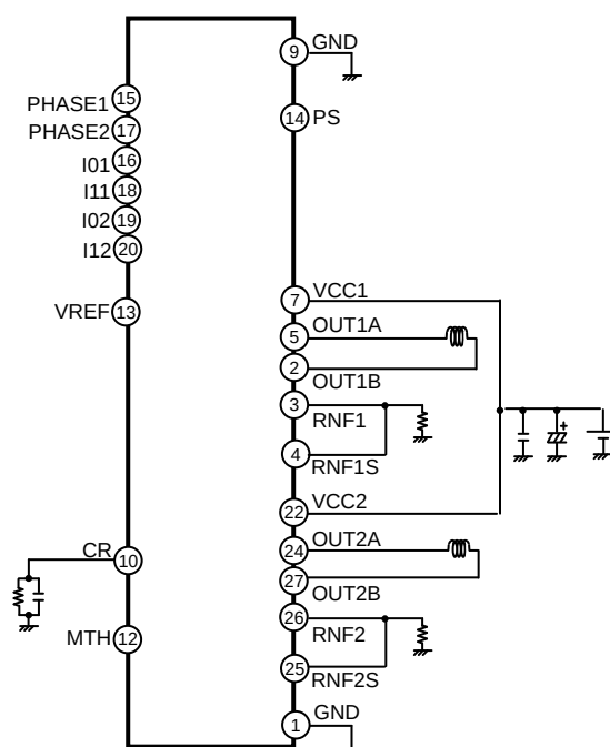
Figure 1. BD68720EFV アプリケーション回路図
