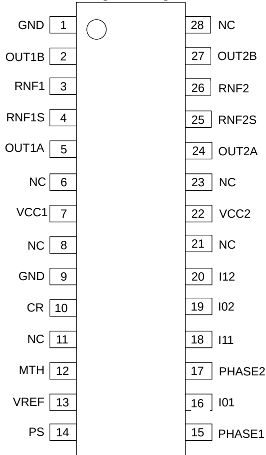
Fig2. 端子配置図
