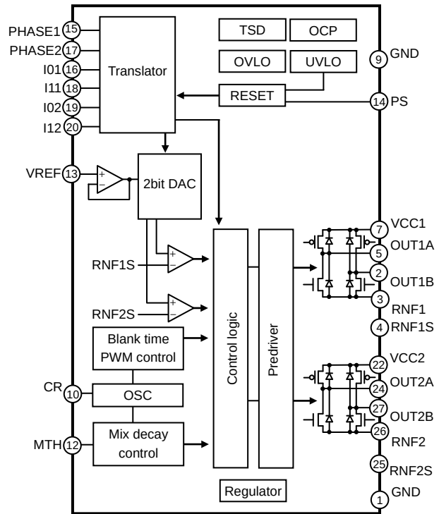
Fig.3 BD68720EFV ブロック図
