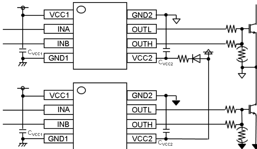
Figure 1. 基本アプリケーション回路 (2ch 使用時)
