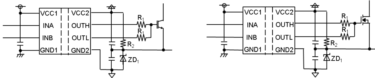
Figure 30. IGBT or MOSFET 駆動時(負電源使用)
