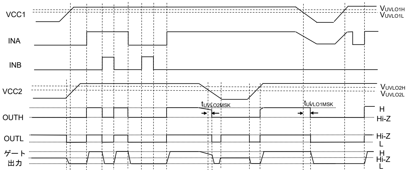
Figure 27. 入出力動作タイミングチャート
