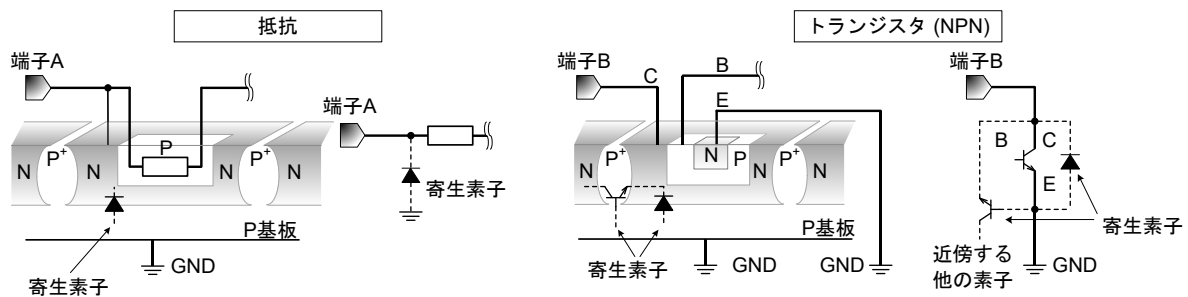
Figure 32. IC 構造例
