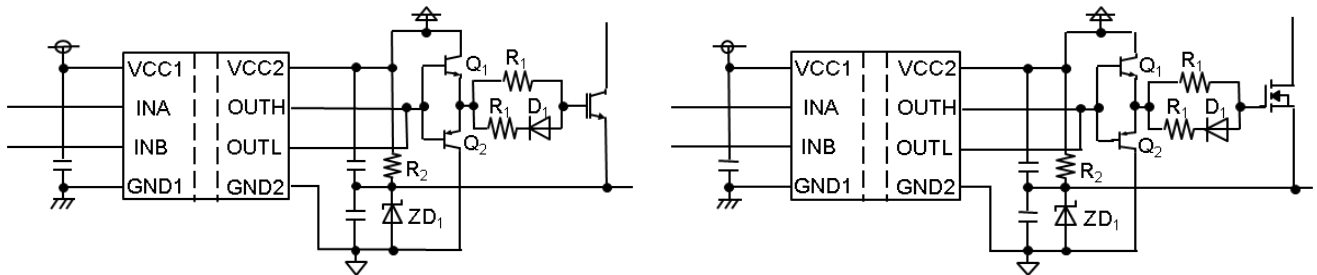
Figure 31. IGBT or MOSFET 駆動時(バッファ回路及び負電源使用)
