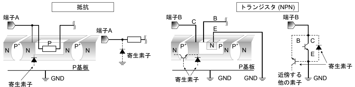
Figure 19. IC 構造例
