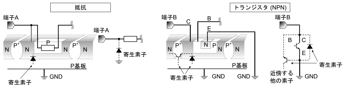
Figure 19. IC 構造例
