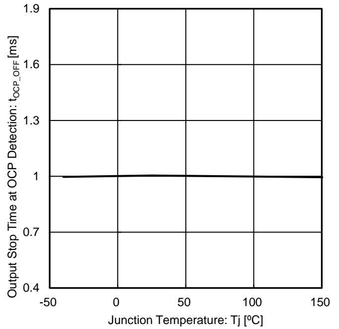
Figure 37. 過電流検出時出力オフ時間 vs 接合部温度
