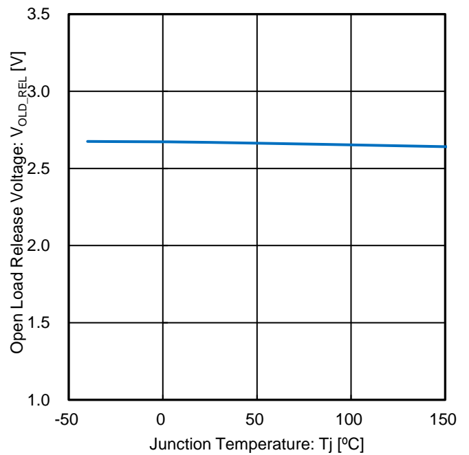
Figure 39. 負荷オープン検出解除電圧 vs 接合部温度
