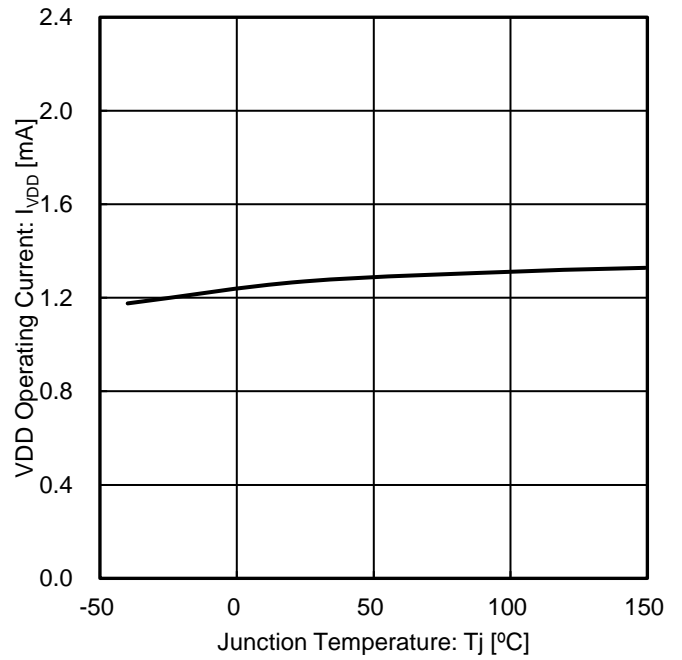
Figure 11. VDD 動作電流 vs 接合部温度
