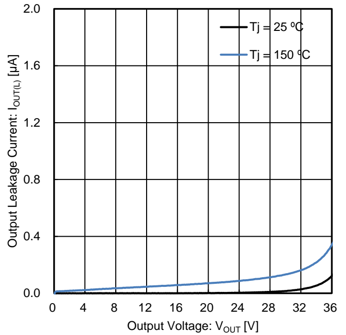
Figure 21. 出力リーク電流 vs 出力電圧
