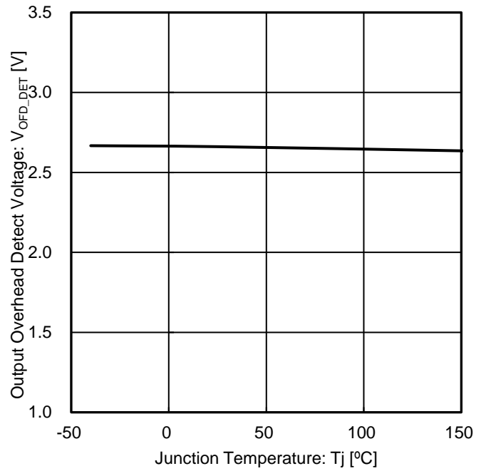
Figure 41. 出力天絡検出検知電圧 vs 接合部温度
