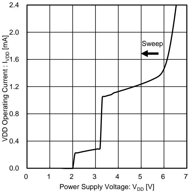
Figure 10. VDD 動作電流 vs 電源電圧
