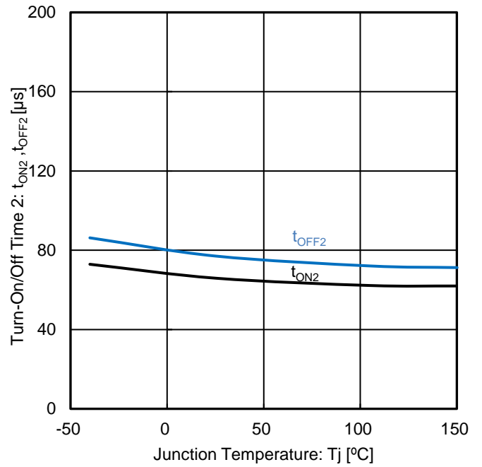
Figure 29. ターンオン/オフ時間 2 vs 接合部温度
