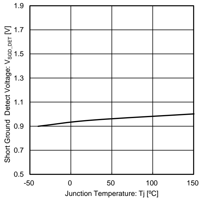
Figure 43. 出力地絡検出検知電圧 vs 接合部温度
