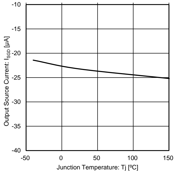
Figure 45. 出力地絡検出動作時出力流出電流 vs 接合部温度
