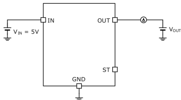
Figure 18、Figure 19 の測定回路図
