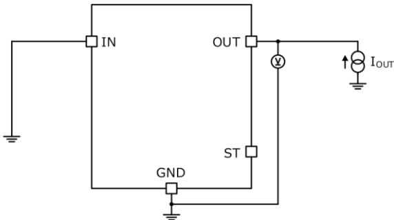
Figure 8、Figure 9 の測定回路図
