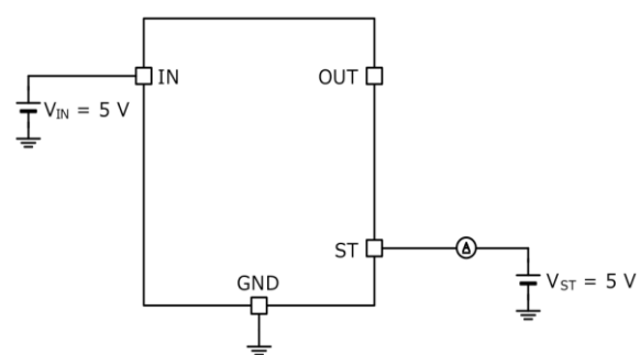
Figure 20 の測定回路図
