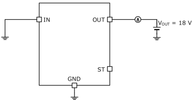
Figure 5 の測定回路図
