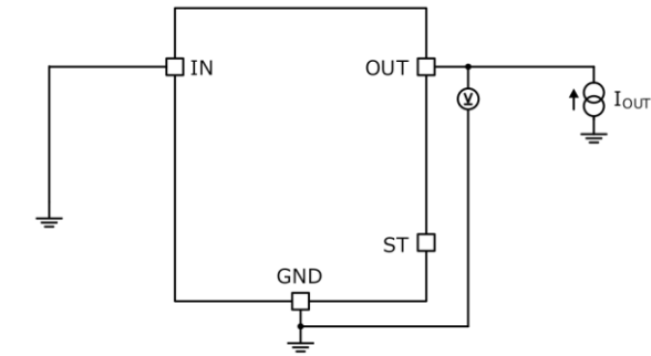
Figure 8、Figure 9 の測定回路図
