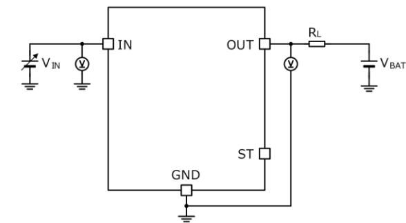
Figure 2 の測定回路図
