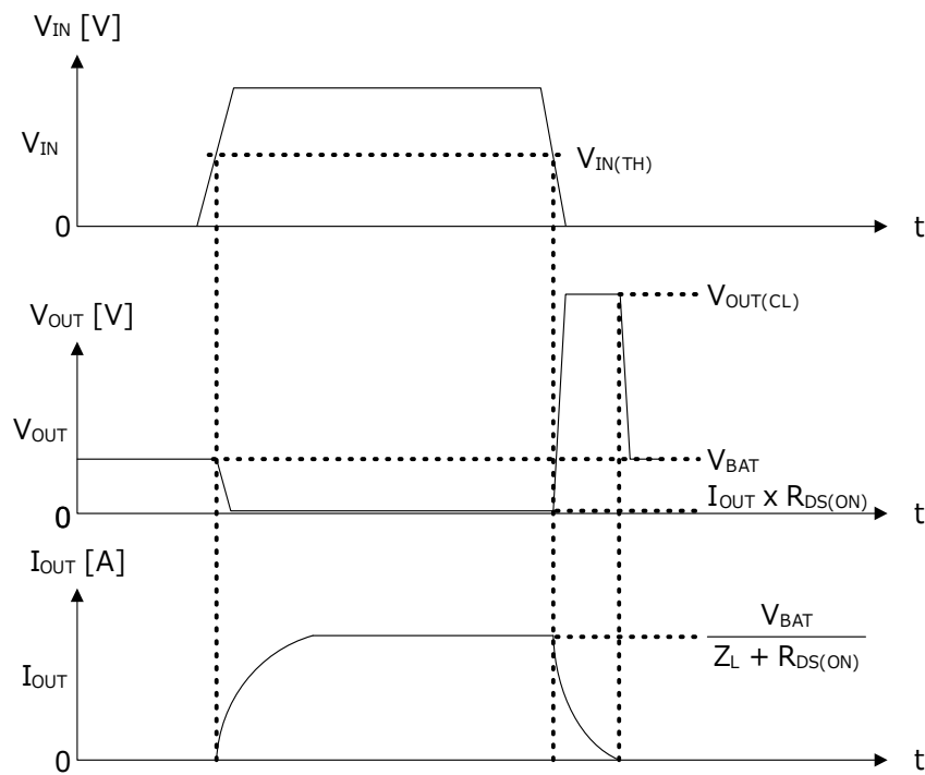
Figure 22. 誘導性負荷時動作
