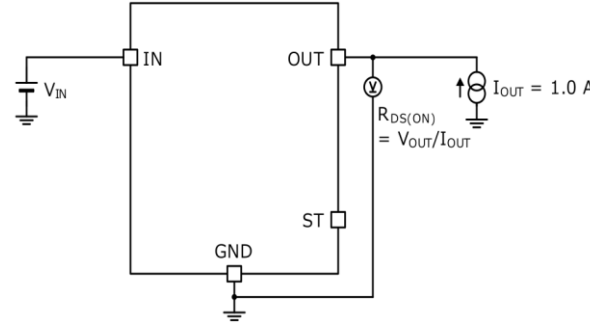
Figure 6、Figure 7 の測定回路図
