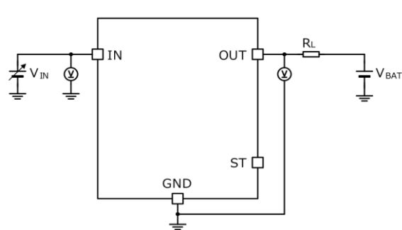
Figure 2 の測定回路図
