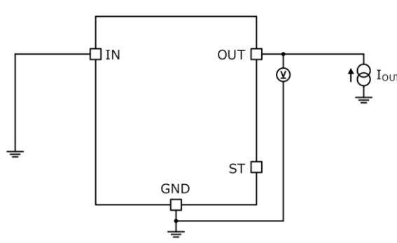
Figure 8、Figure 9 の測定回路図
