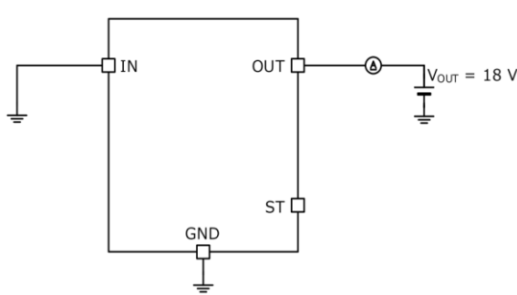
Figure 5 の測定回路図
