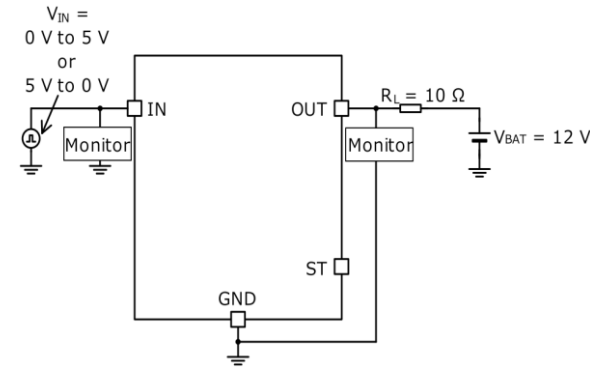
Figure 10、Figure 11、Figure 12、Figure 13、Figure 14、 Figure 15、Figure 16、Figure 17 の測定回路図
