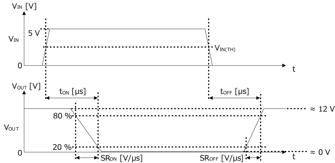
Figure 21. ターンオン時間、ターンオフ時間、スループートの定義
