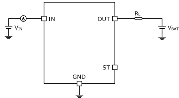
Figure 3、Figure 4 の測定回路図
