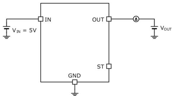
Figure 18、Figure 19 の測定回路図
