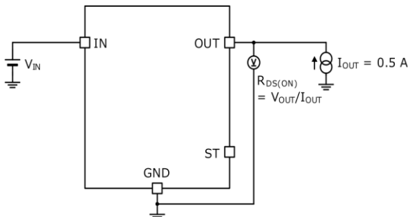
Figure 6、Figure 7 の測定回路図
