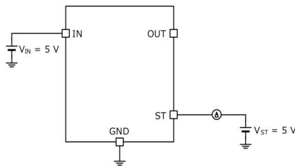
Figure 20 の測定回路図
