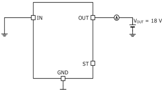
Figure 5 の測定回路図
