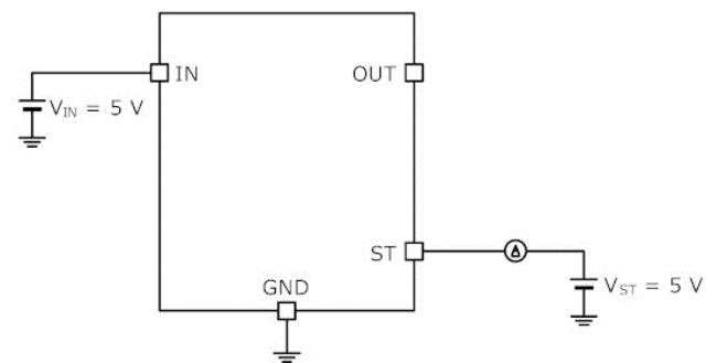
Figure 20 の測定回路図
