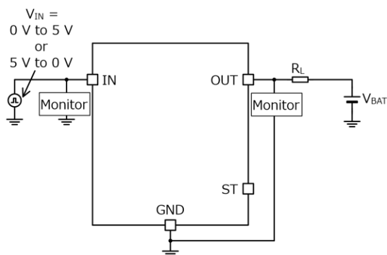
Figure 10、Figure 11、Figure 12、Figure 13、Figure 14、 Figure 15、Figure 16、Figure 17 の測定回路図
