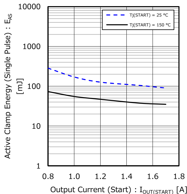
Figure 1. アクティブクランプ耐量 (Single Pulse) vs 出力電流 (Start)
