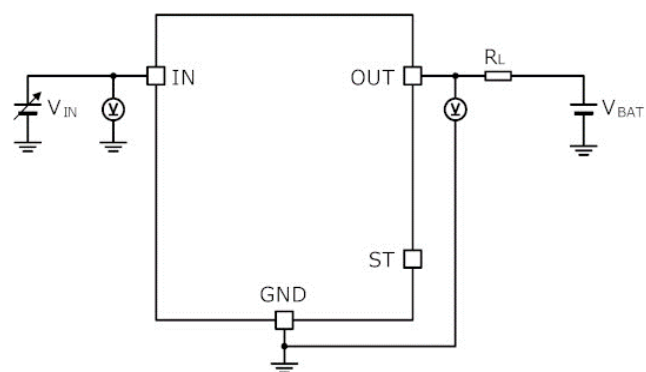
Figure 2 の測定回路図
