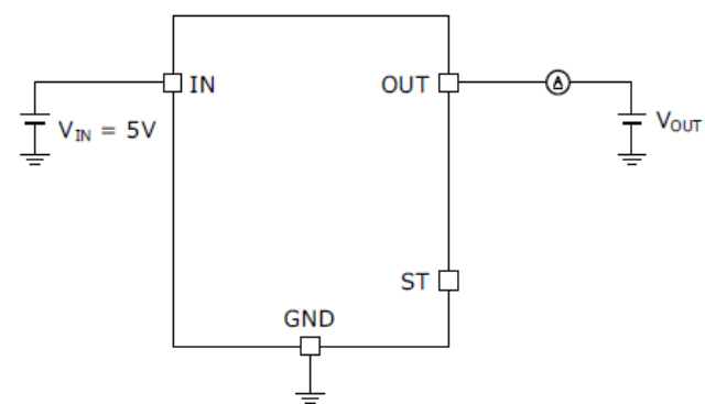
Figure 18、Figure 19 の測定回路図
