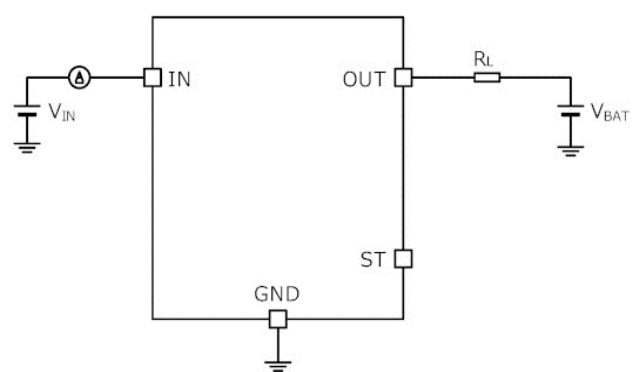
Figure 3、Figure 4 の測定回路図
