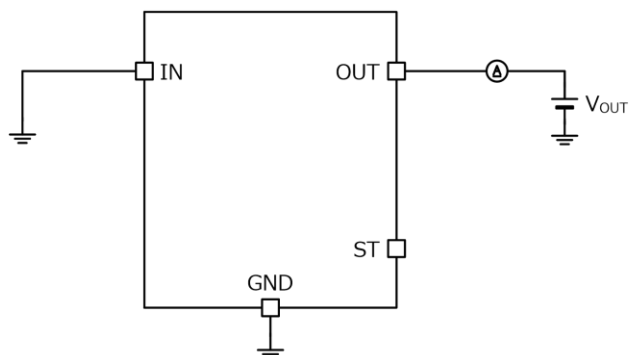
Figure 5 の測定回路図
