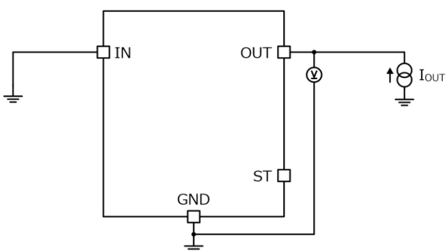
Figure 8、Figure 9 の測定回路図
