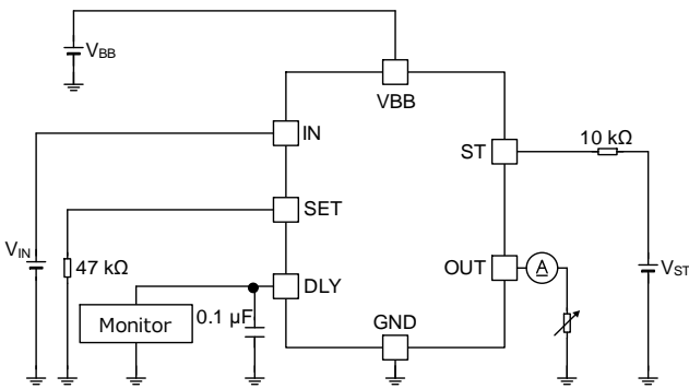
Figure 31. 固定過電流制限値 可変過電流制限値
