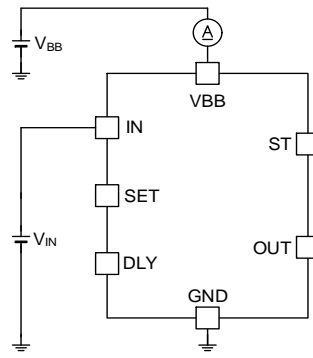
Figure 26. 動作時電流
