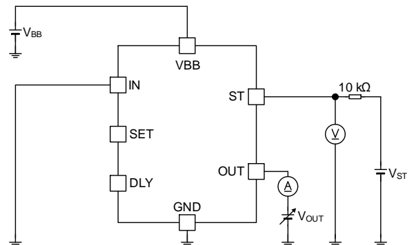
Figure 32. 負荷オープン検出電圧 負荷オープン検出シンク電流
