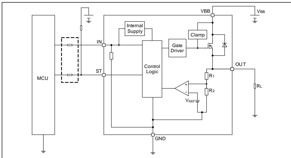
Figure 40. MCU I/O 保護
