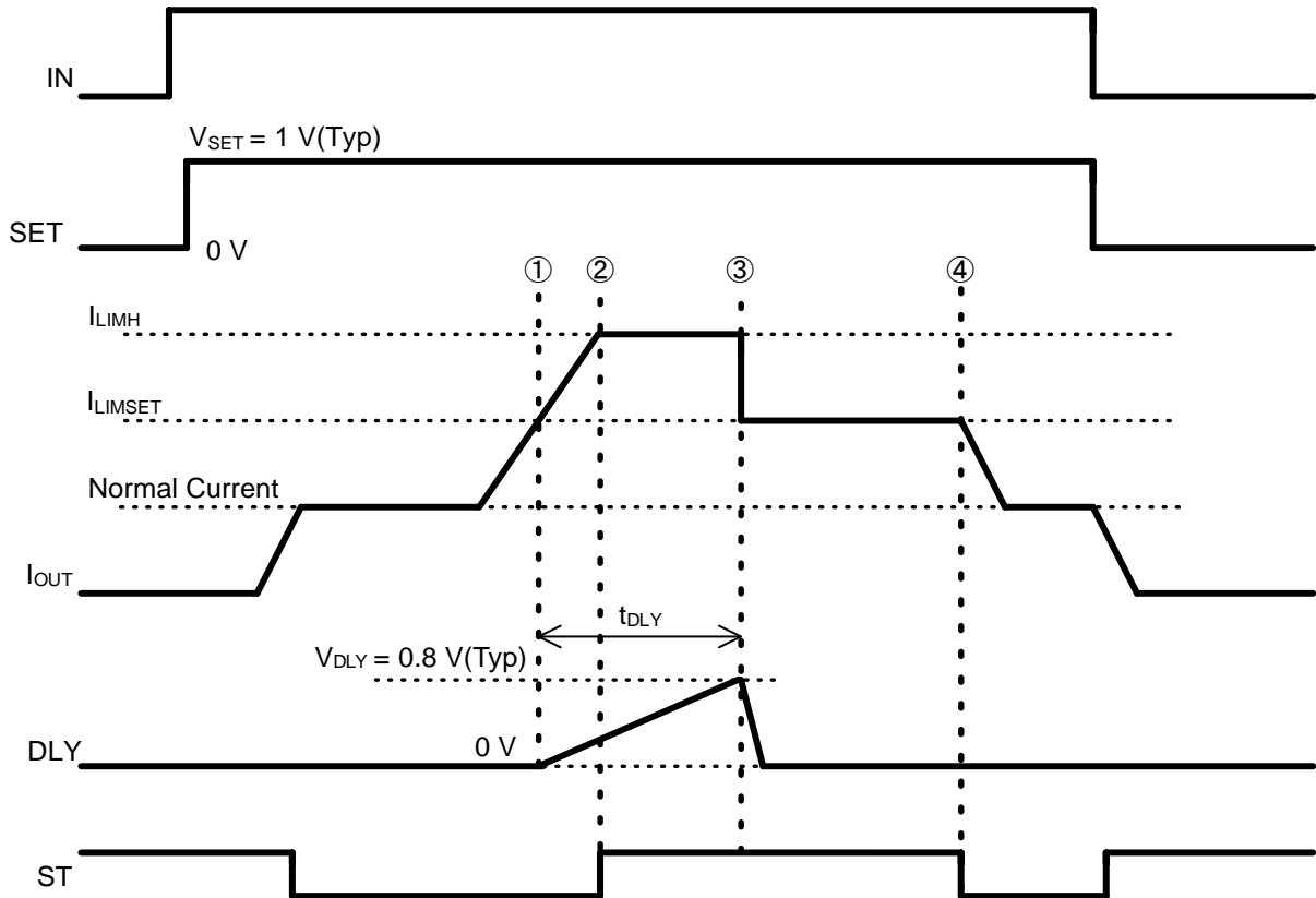
Figure 34. 過電流が流れた場合のタイミングチャート
