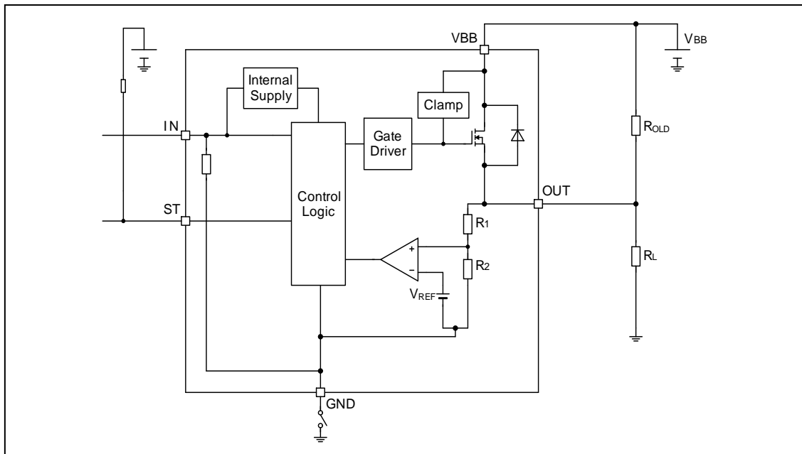
Figure 39. GND オープン保護 ブロック図
