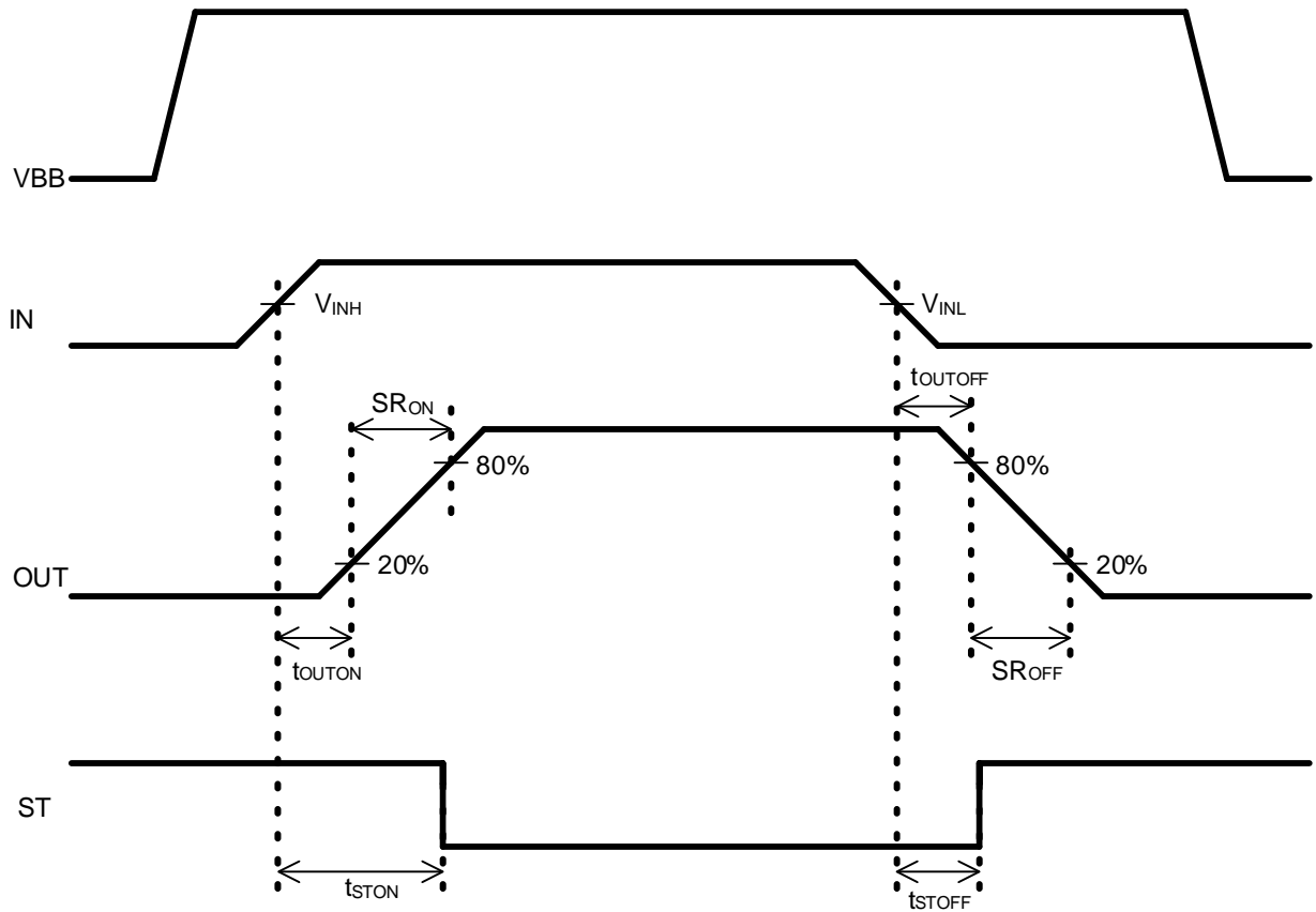
Figure 33. タイミングチャート
