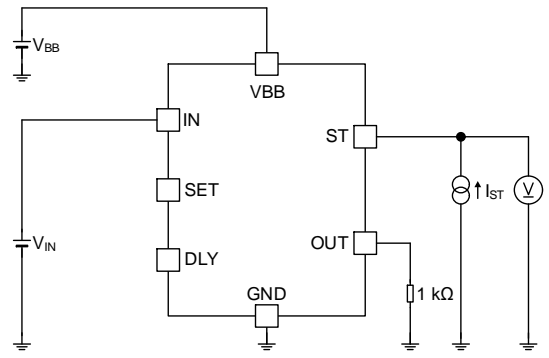
Figure 30. 診断出力 Low 電圧
