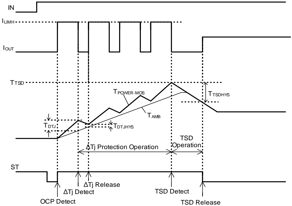
Figure 38. 過熱保護・ \Delta T_j 保護 タイミングチャート
