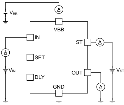
Figure 25. 非動作時電流 Low レベル入力電流 出力リーク電流 診断出力リーク電流
