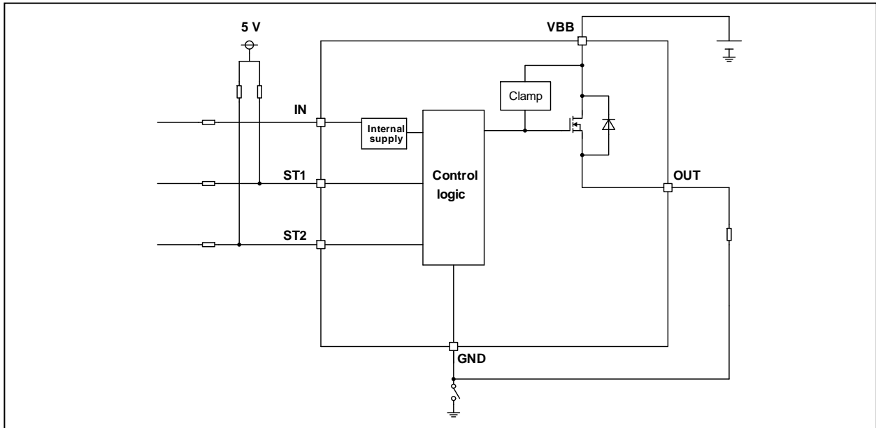
Figure 37. GND オープン保護 ブロック図
