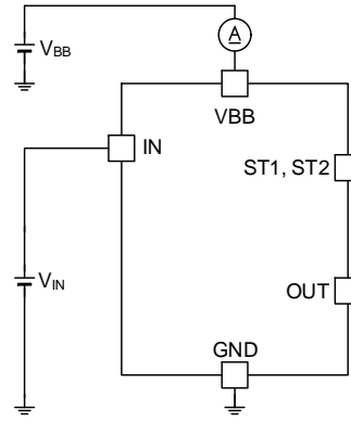
Figure 26. 動作時電流
