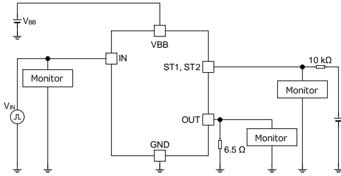
Figure 29. オン時出力スルーレート オフ時出力スルーレート オン時伝播遅延時間 オフ時伝播遅延時間 診断出力オン時伝播遅延時間 診断出力オフ時伝播遅延時間
