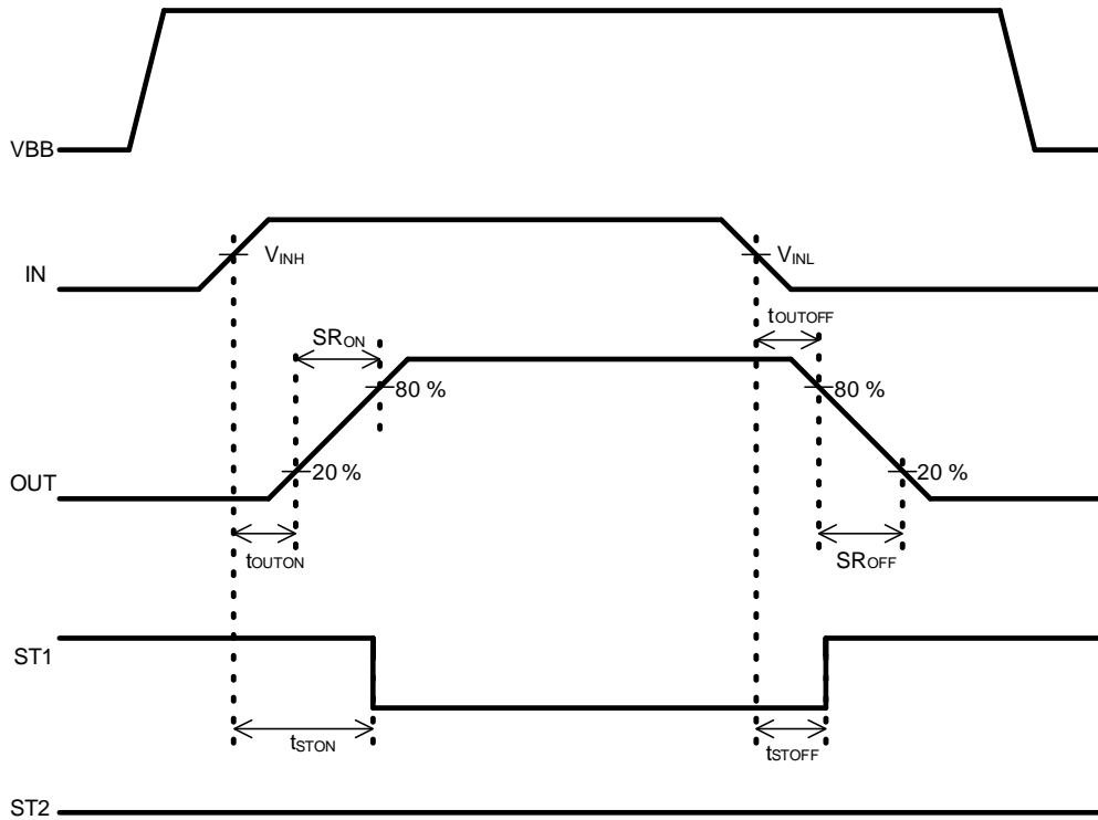
Figure 34. タイミングチャート
