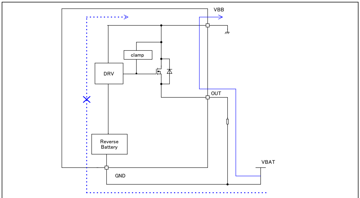
Figure 38. バッテリー逆接続 ブロック図
