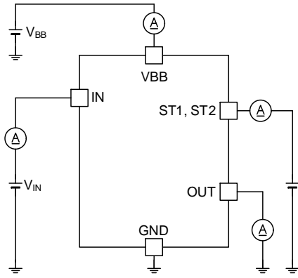
Figure 25. 非動作時電流 Low レベル入力電流 出力リーク電流 診断出力リーク電流
