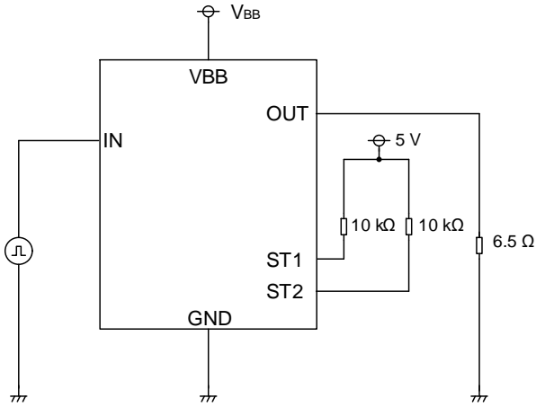
Figure 32. スイッチングタイム測定図
