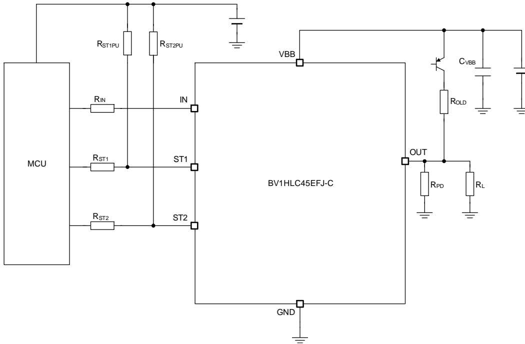
Figure 40. 応用回路図
