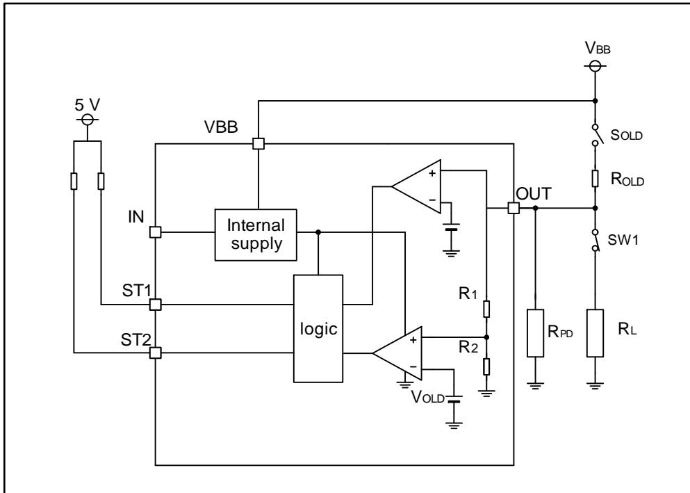
Figure 36. 負荷オープン検出 ブロック図
