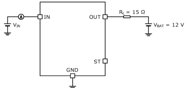
Figure 15、Figure 16 の測定回路図
