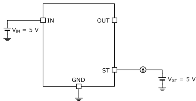
Figure 20 の測定回路図
