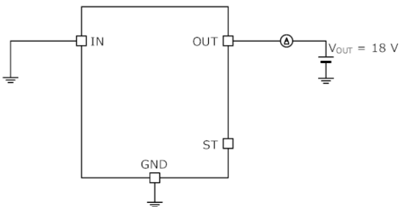
Figure 5 の測定回路図
