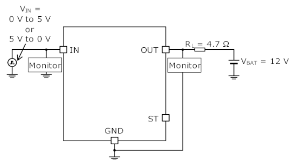
Figure 10、Figure 11、Figure 12、Figure 13、 Figure 14、Figure 15、Figure 16、Figure 17 の測定回路図
