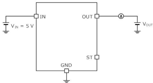
Figure 18、Figure 19 の測定回路図
