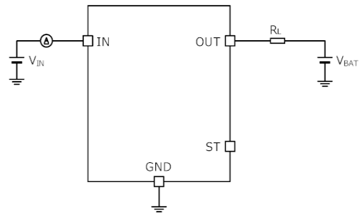
Figure 3、Figure 4 の測定回路図
