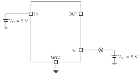
Figure 20 の測定回路図
