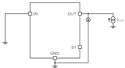
Figure 8、Figure 9 の測定回路図
