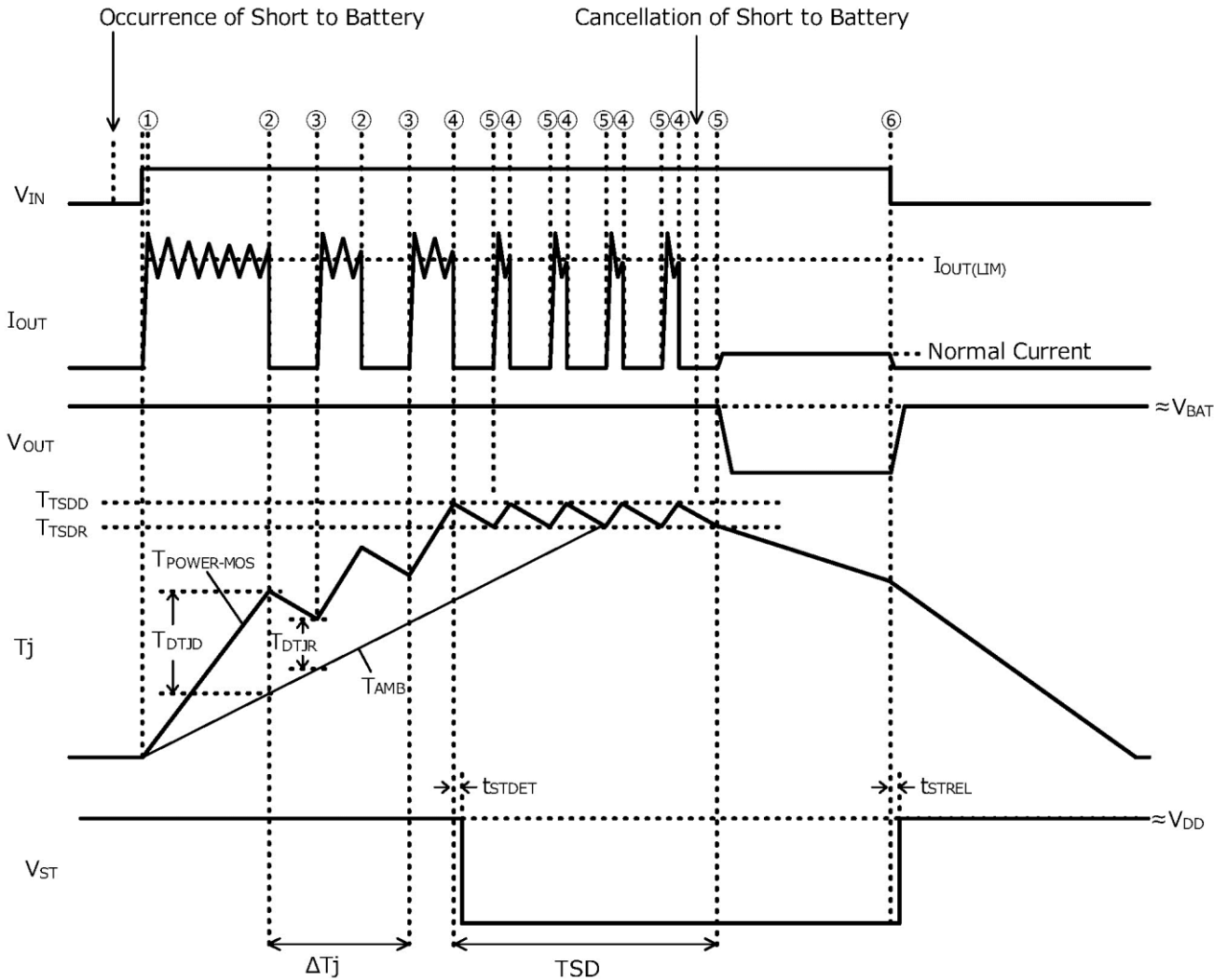
Figure 23. OUT 端子短絡時のタイミングチャート
