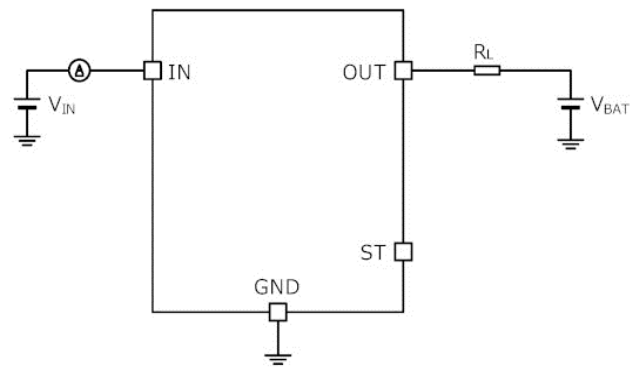
Figure 3、Figure 4 の測定回路図
