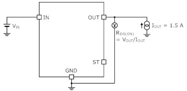
Figure 6、Figure 7 の測定回路図
