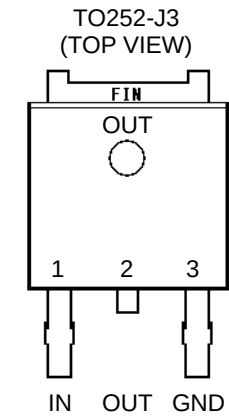
Figure 2. 端子配置図
