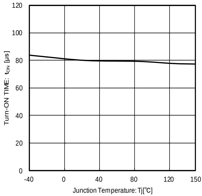
Figure 15. ターンオン時間 vs ジャンクション温度
