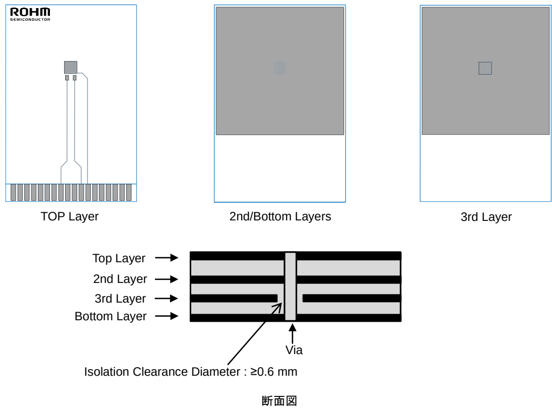
Figure 6. PCB レイアウト 4 層 (2s2p)
