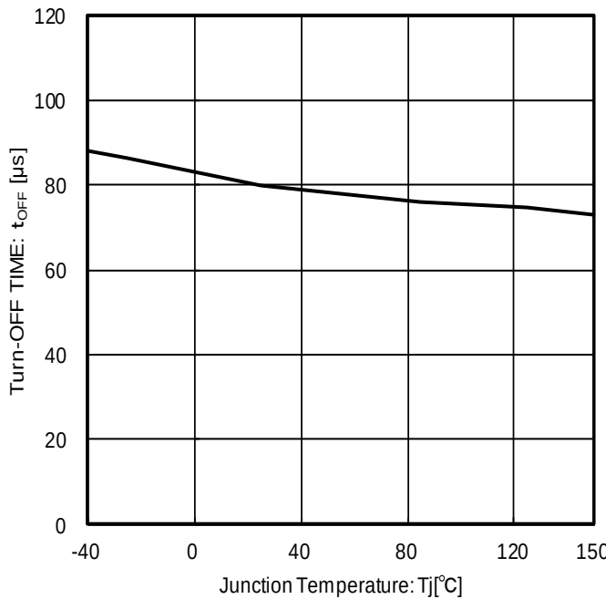
Figure 16. ターンオフ時間 vs ジャンクション温度
