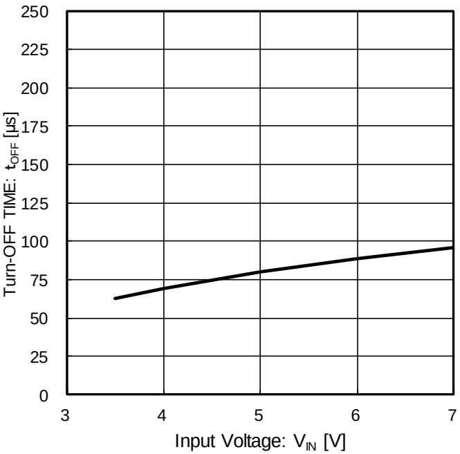
Figure 14. ターンオフ時間 vs 入力電圧
