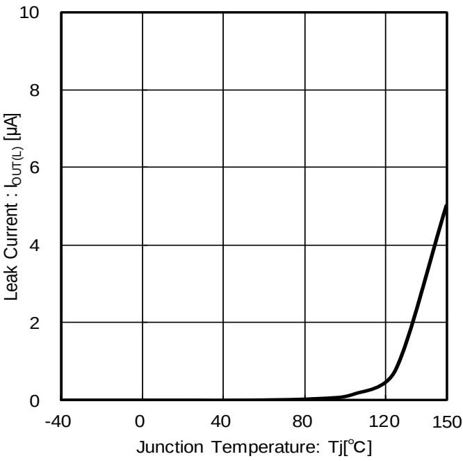
Figure 12. リーク電流 vs ジャンクション温度
