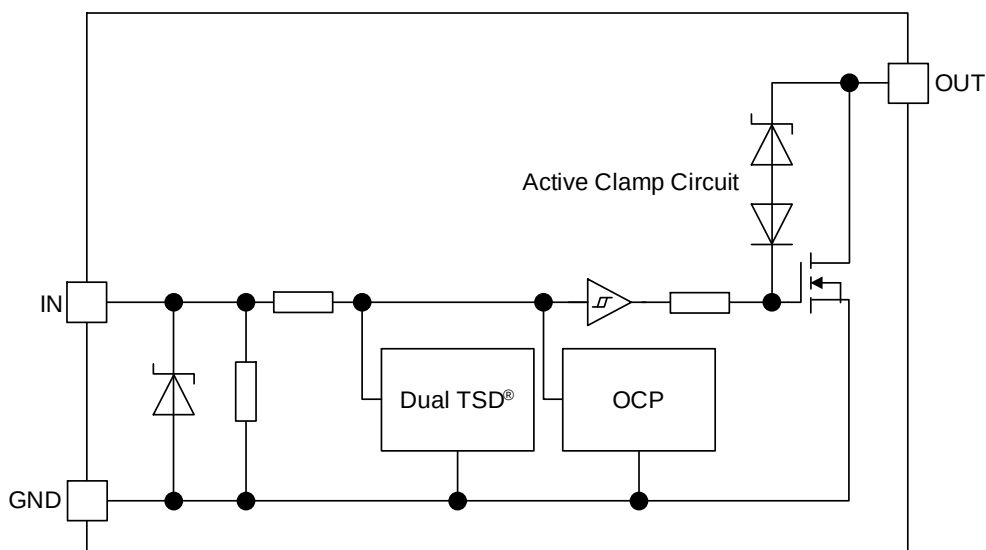
Figure 1. ブロック図
