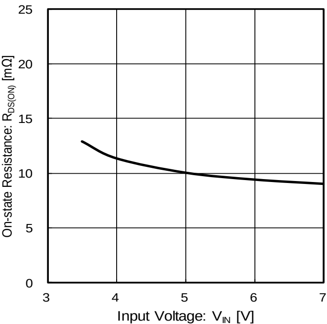
Figure 10. オン抵抗 vs 入力電圧
