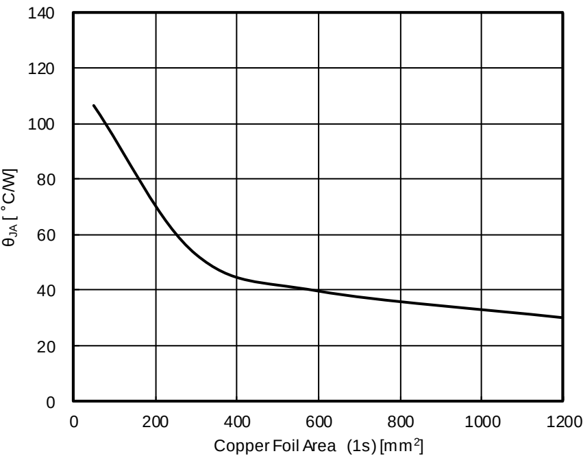
Figure 8. 熱抵抗
