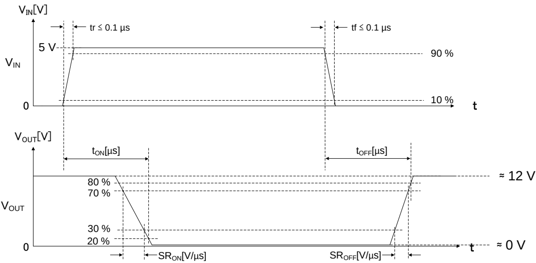
Figure 27. ターンオン時間、ターンオフ時間、スルーレートの定義
