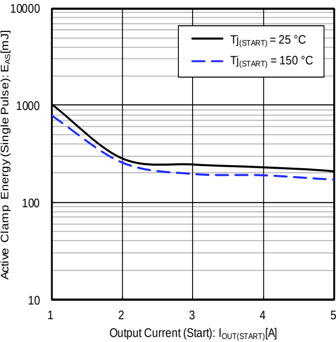
Figure 25. アクティブクランプ耐量 (Single Pulse) vs 出力電流 (Start)
