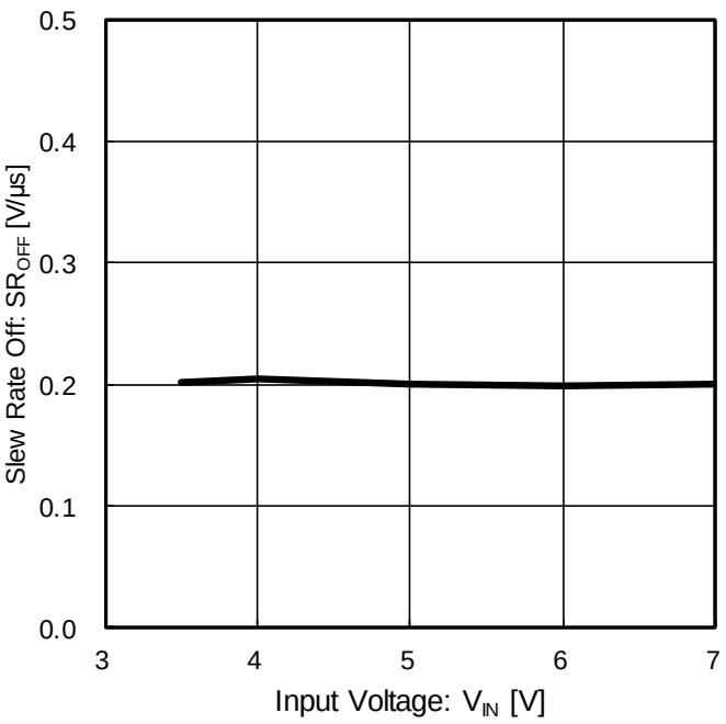
Figure 18. スルーレート（オフ） vs 入力電圧
