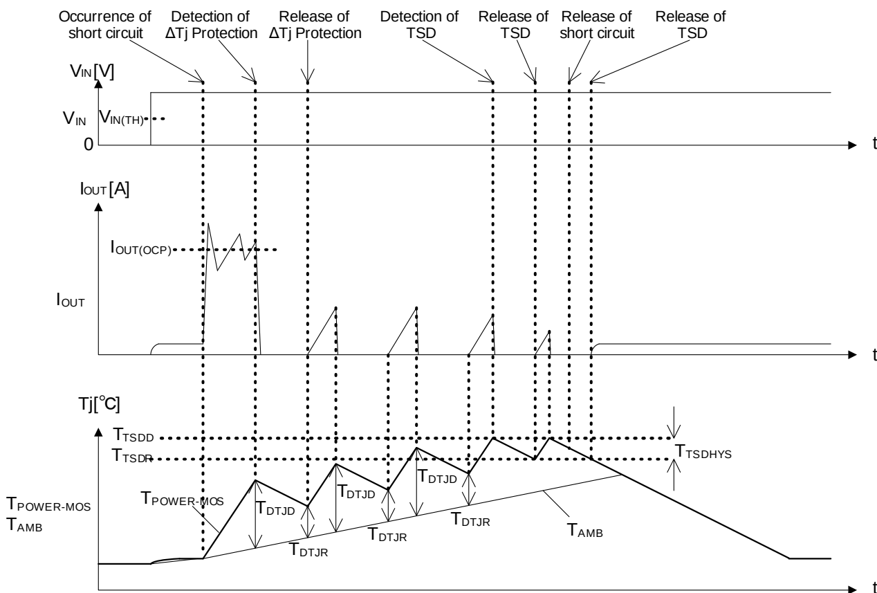
Figure 28. 出力端子ショート時の動作
