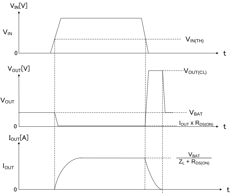
Figure 26. 誘導性負荷時動作
