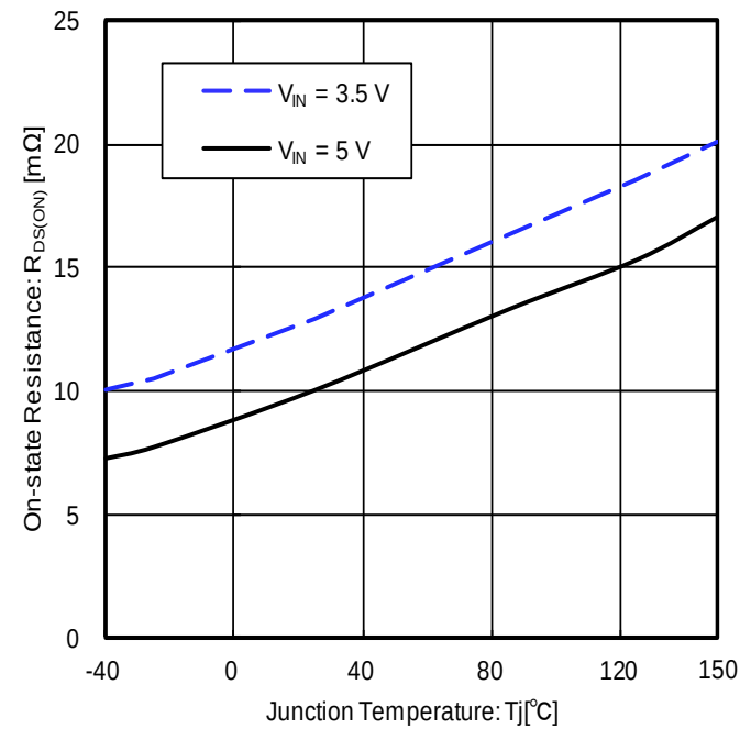
Figure 11. オン抵抗 vs ジャンクション温度
