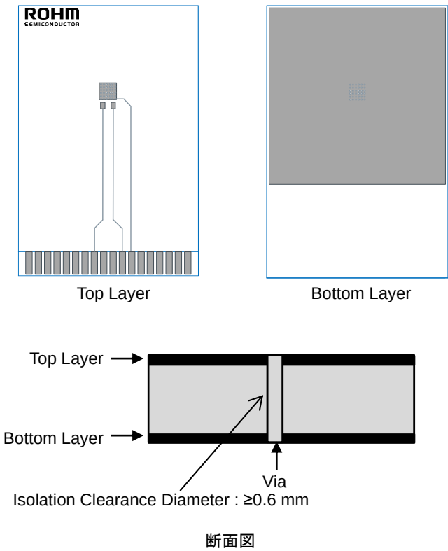
Figure 5. PCB レイアウト 2 層 (2s)
