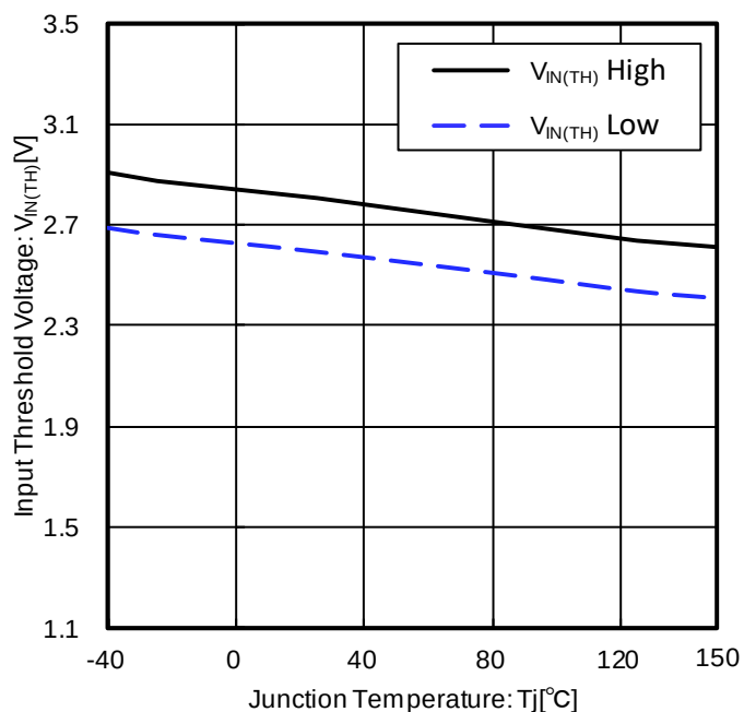
Figure 21. 入カスレッシュOLD電圧 vs ジャンクション温度
