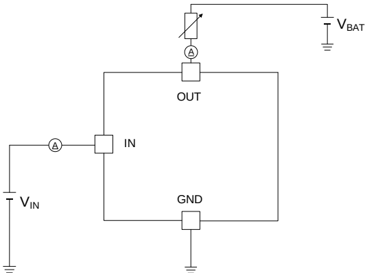
Figure 24 の回路図
