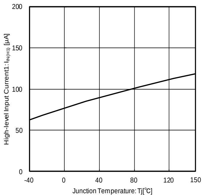
Figure 23. ハイレベル入力電流 1 (通常時) vs ジャンクション温度
