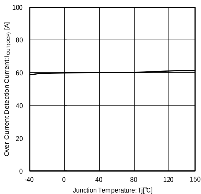
Figure 24. 過電流検出電流 vs ジャンクション温度
