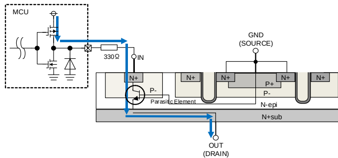
Figure 29. 出力負電流経路(パワーMOS オン時)
