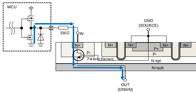
Figure 30. 出力負電流経路(パワーMOS オフ時)
