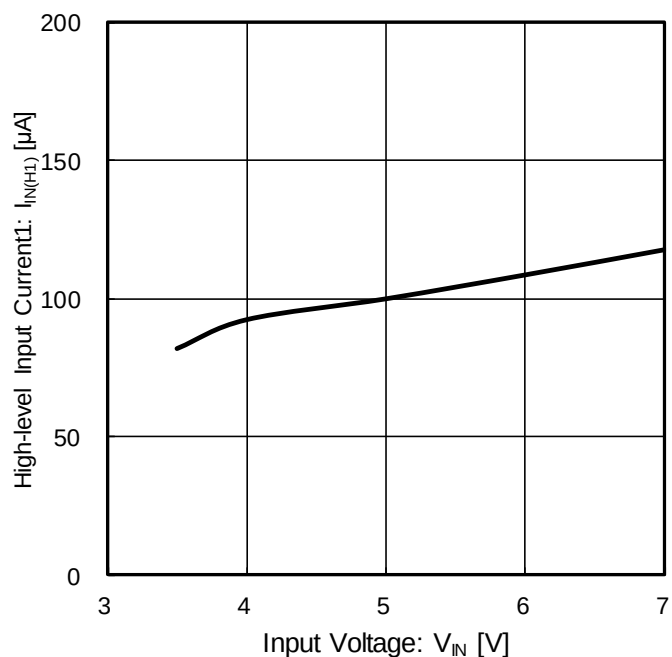
Figure 22. ハイレベル入力電流 1 (通常時) vs 入力電圧
