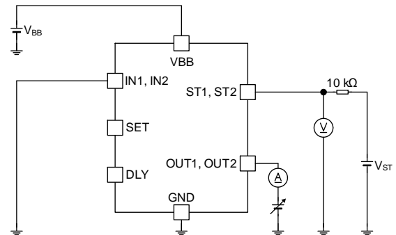
Figure 31. 負荷オープン検出電圧 負荷オープン検出シンク電流
