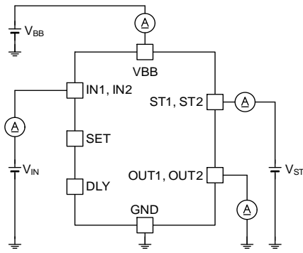
Figure 24. 非動作時電流 Low レベル入力電流 出力リーク電流 診断出力リーク電流
