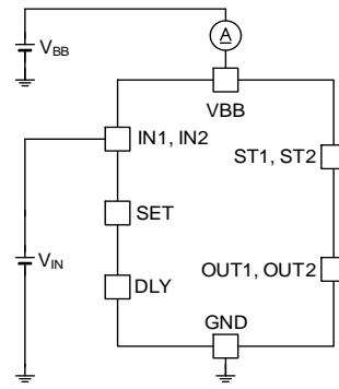
Figure 25. 動作時電流
