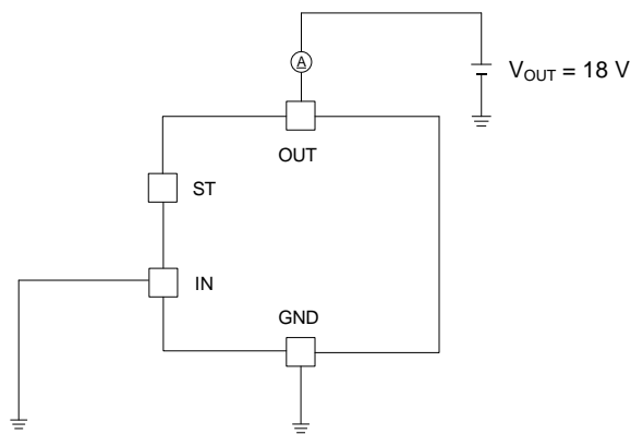
Figure 13 の測定回路図
