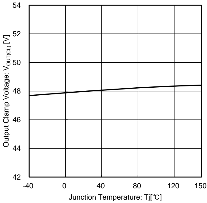
Figure 10. 出カクランプ電圧 vs ジャンクション温度
