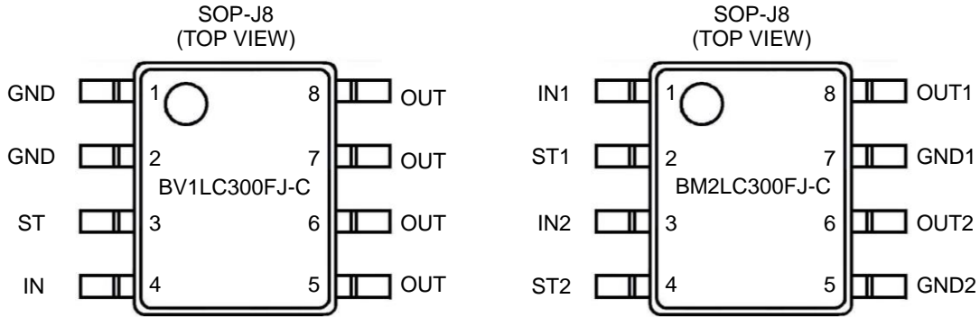
Figure 2. 端子配置図
