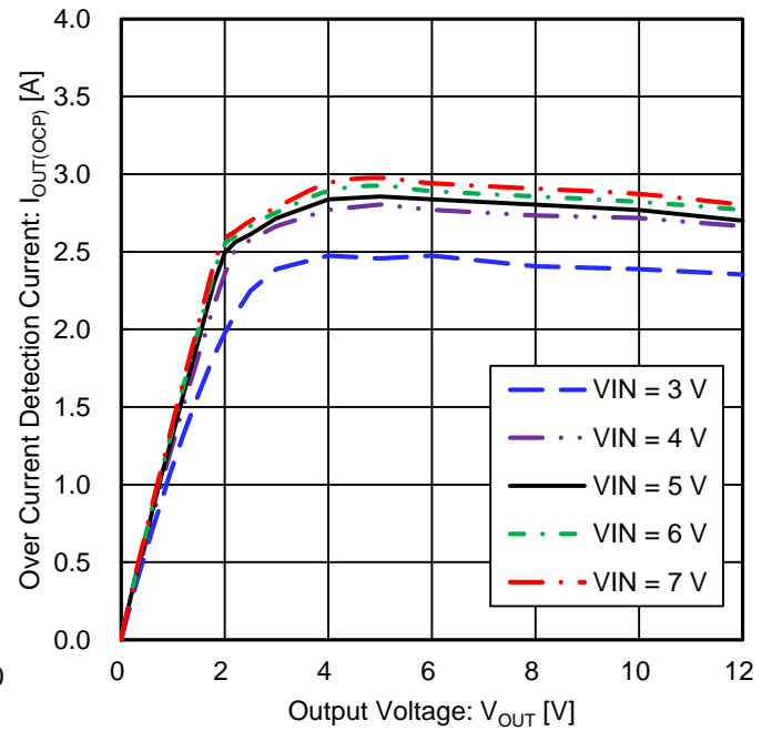
Figure 25. 過電流検出電流 vs 出力電圧
