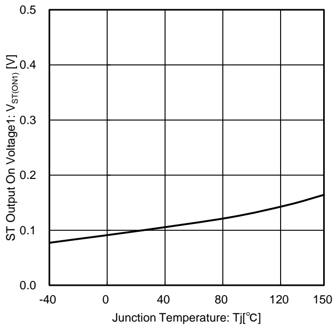
Figure 28. ST 出力オン電圧 1 vs ジャンクション温度
