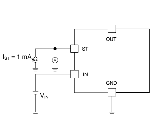
Figure 28 の測定回路図
