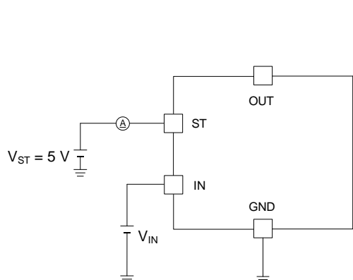
Figure 30 の測定回路図
