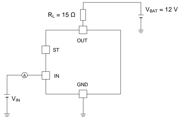
Figure 23、24 の測定回路図
