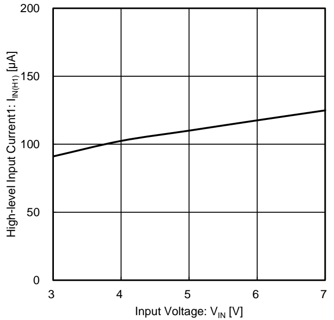
Figure 23. ハイレベル入力電流 1 (通常時) vs 入力電圧
