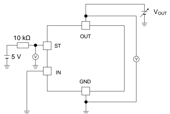
Figure 27 の測定回路図
