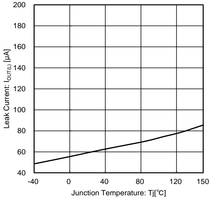
Figure 13. リーク電流 vs ジャンクション温度
