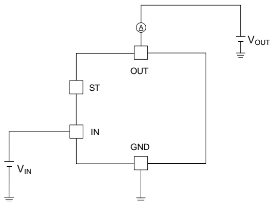
Figure 25、26 の回路図
