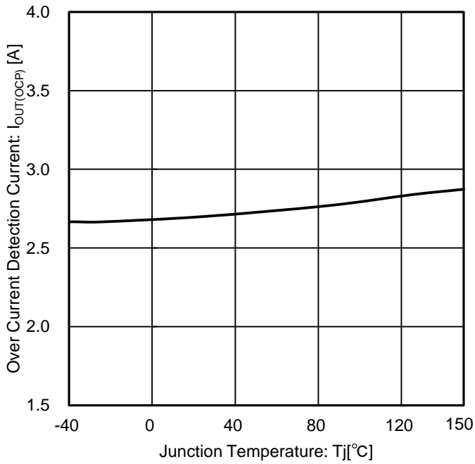
Figure 26. 過電流検出電流 vs ジャンクション温度
