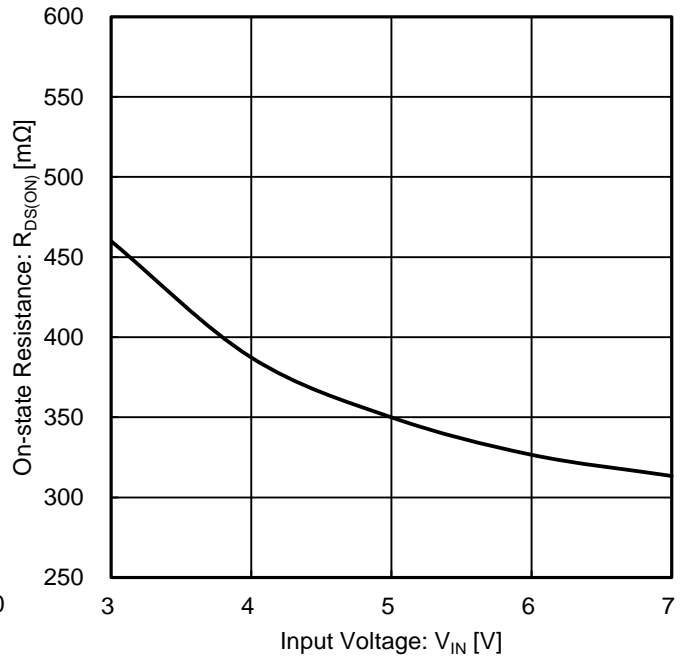
Figure 11. オン抵抗 vs 入力電圧
