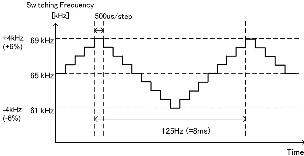
Figure 7. 周波数ホッピング機能
