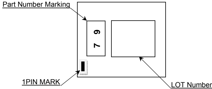
SSOP6(TOP VIEW)
