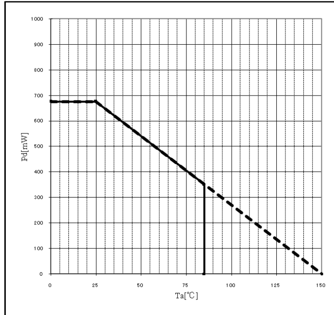
Figure 28 SSOP6 熱軽減特性
