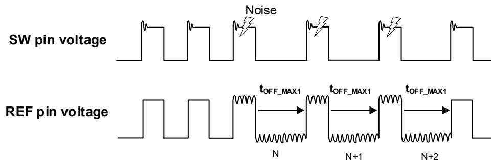
Figure 10. 3-step MAXOFF
