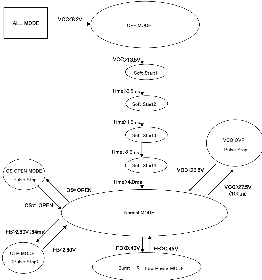
Figure 31. 各状態遷移図(VCCOVP 自己復帰)
