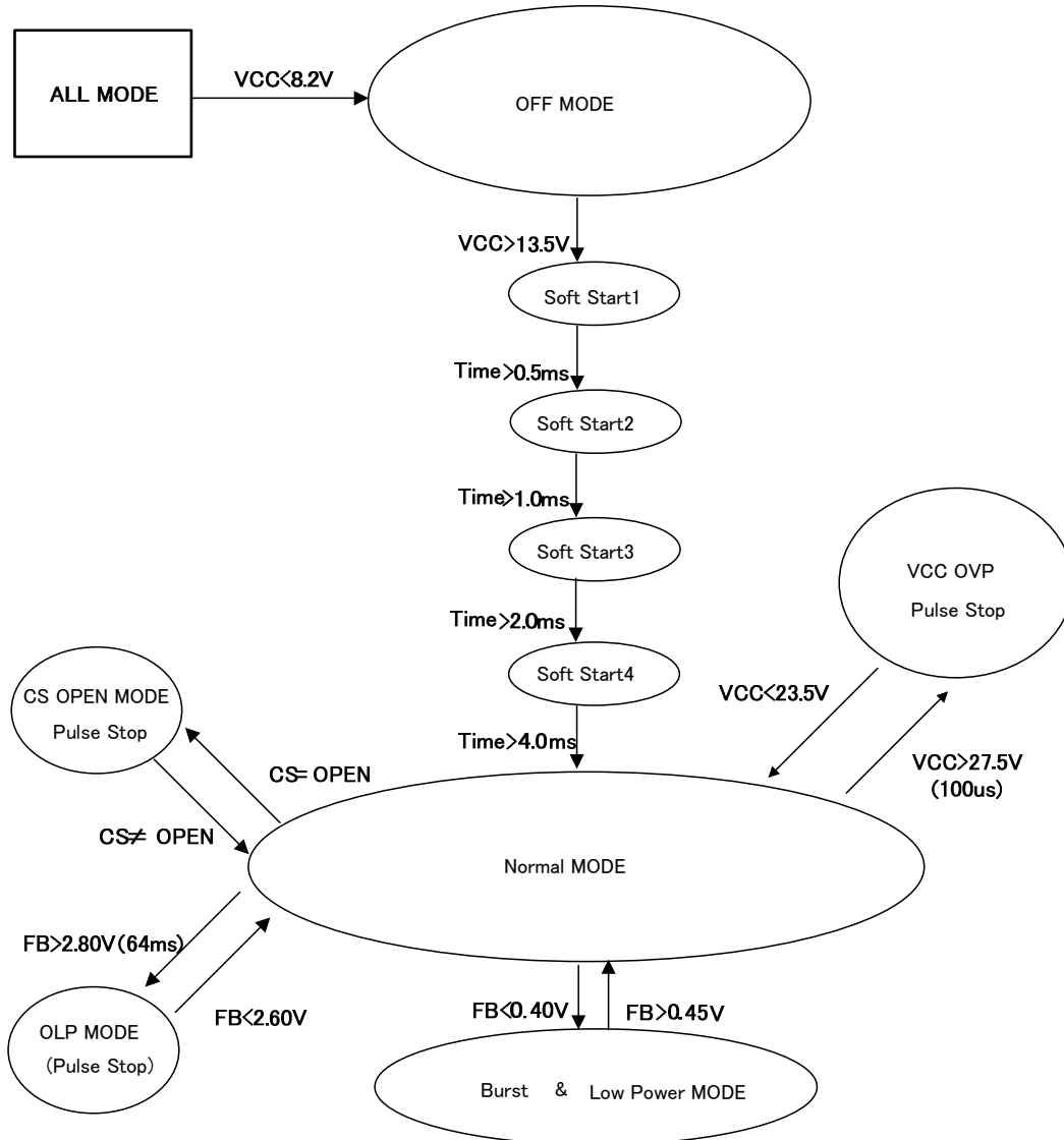
Figure 31. 各状態遷移図(VCCOVP ラッチ)
