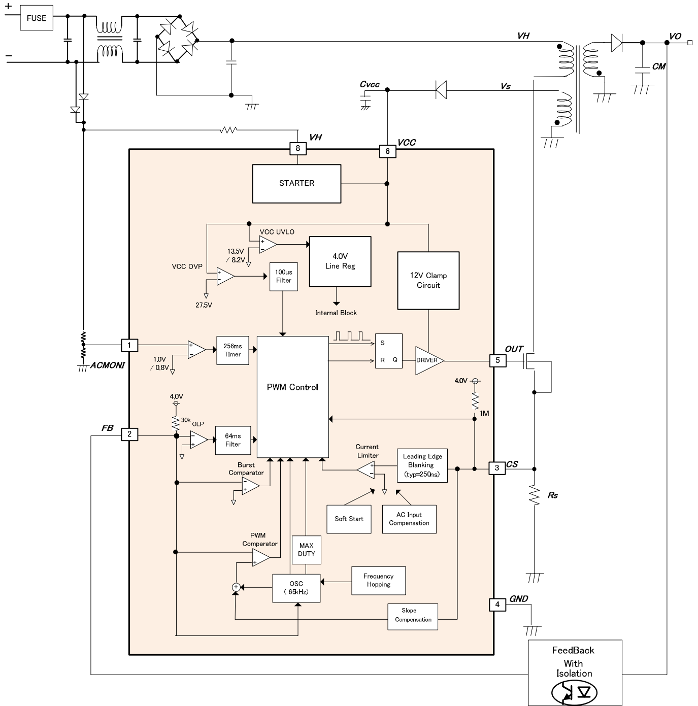
Figure 3. ブロック図
