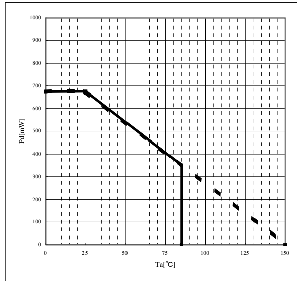
Figure 32. 熱軽減特性
