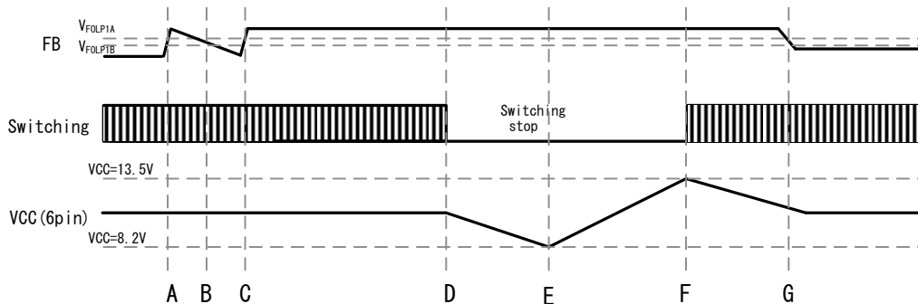
Figure 26. 過負荷保護動作
