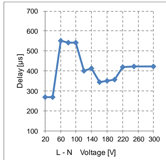
Figure 18. Delay vs L - N Voltage (通常整流時の参考データ)
