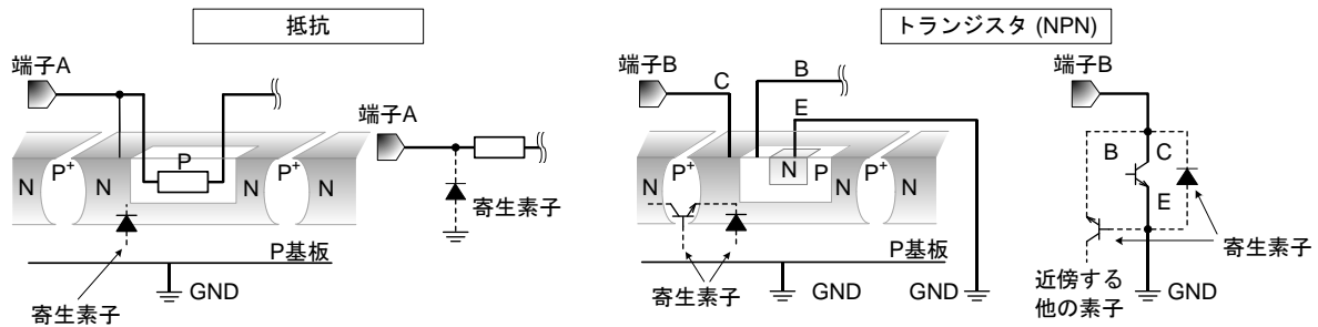
Figure 23. IC 構造例
