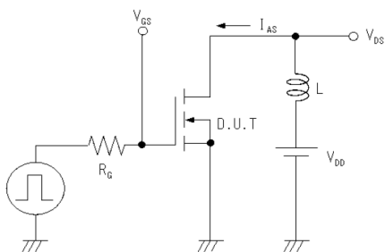
アバランシェエネルギー測定回路
