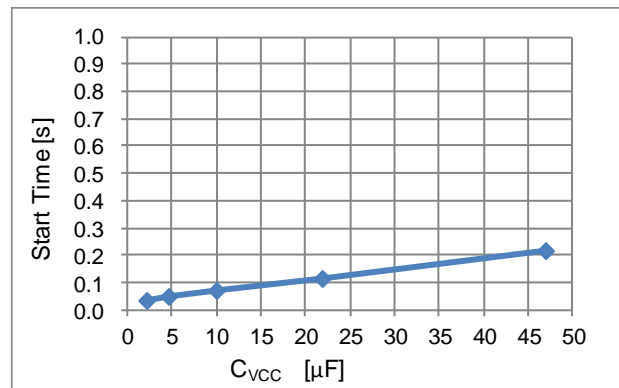
Figure 6. 起動時間 (参考値)
