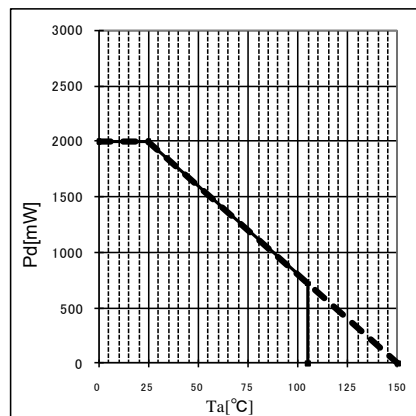
Figure 18. DIP7K 熱軽減特性
