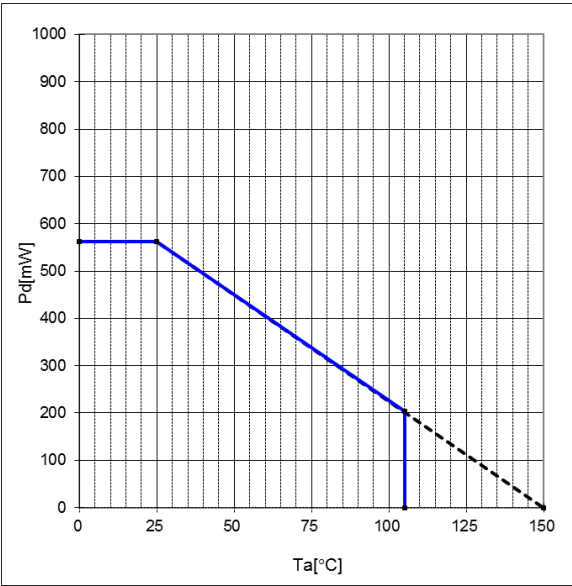
Figure 15. 熱軽減特性
