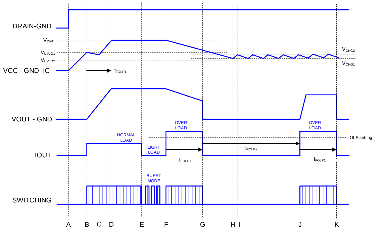
Figure 3. 起動シーケンス タイムチャート
