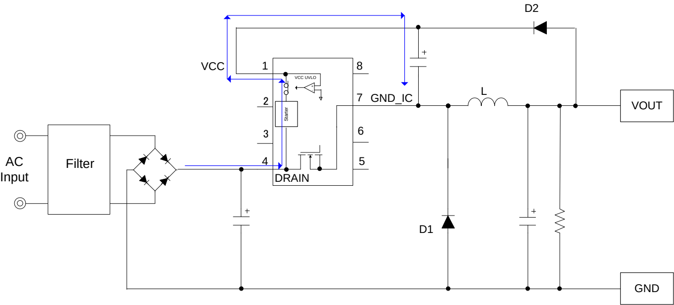
Figure 5. 起動回路
