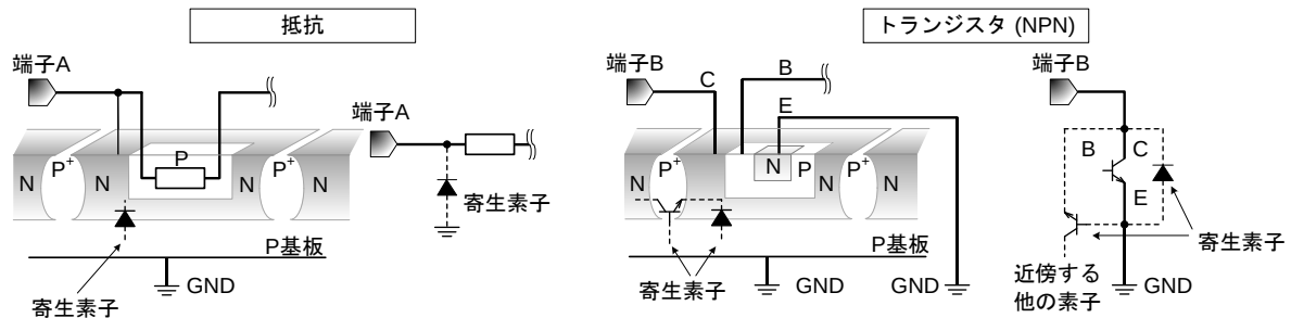
Figure 29. IC 構造例
