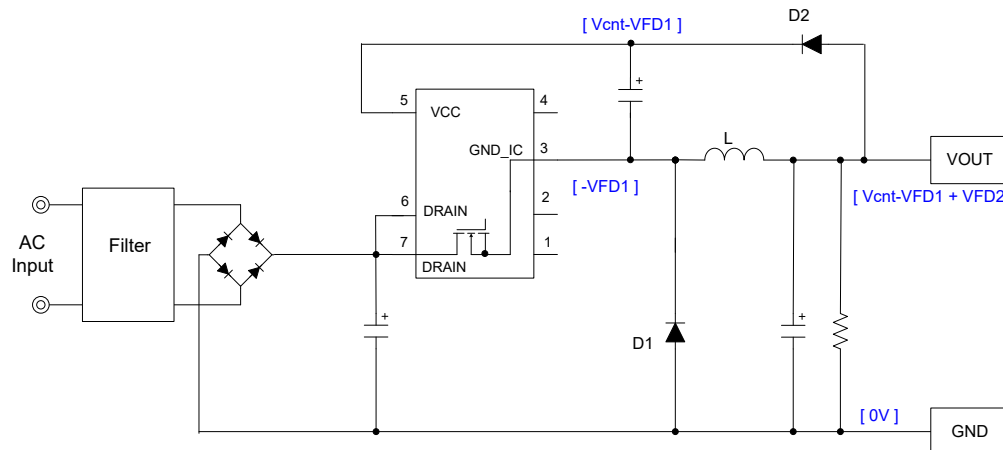
Figure 8. バックコンバータ回路 (MOSFET オフ時)
