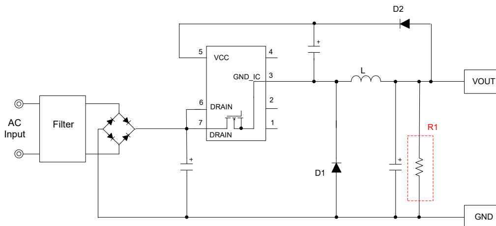
Figure 9. 軽負荷時 電圧持ち上がり対策回路
