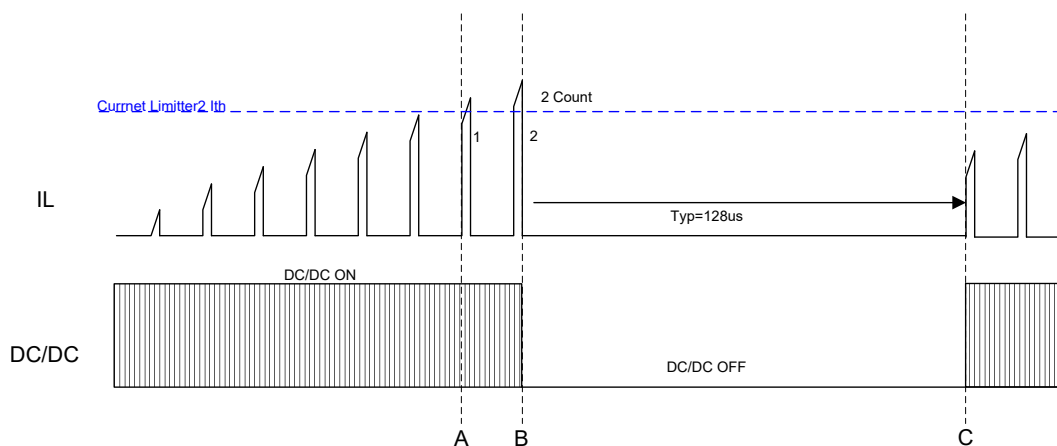
Figure 12. スイッチング周波数 状態遷移
