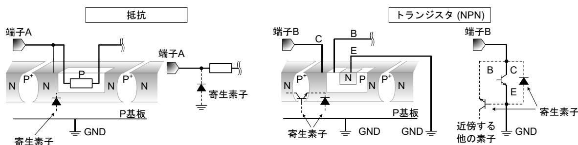
Figure モノリシック IC 構造例
