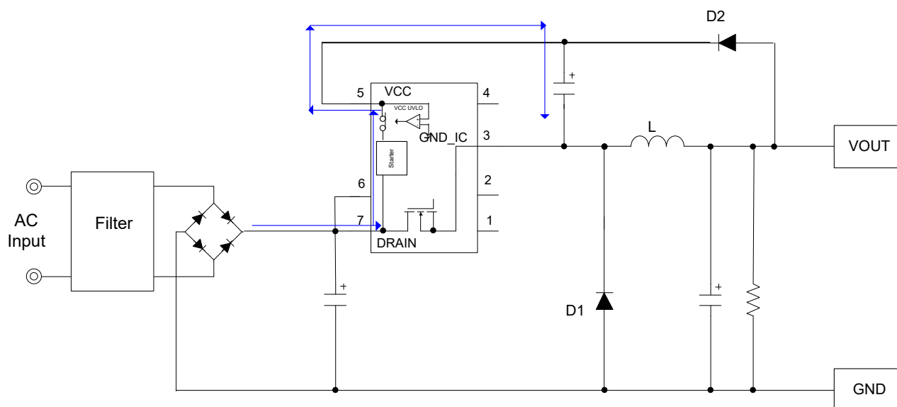
Figure 5. 起動回路
