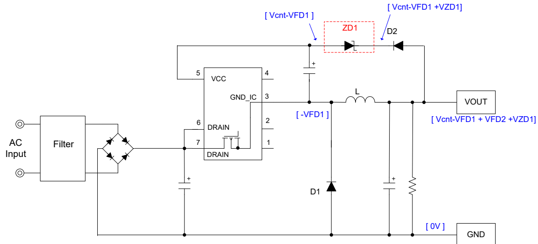
Figure 10. バックコンバータ出力可変回路 (MOSFET オフ時)
