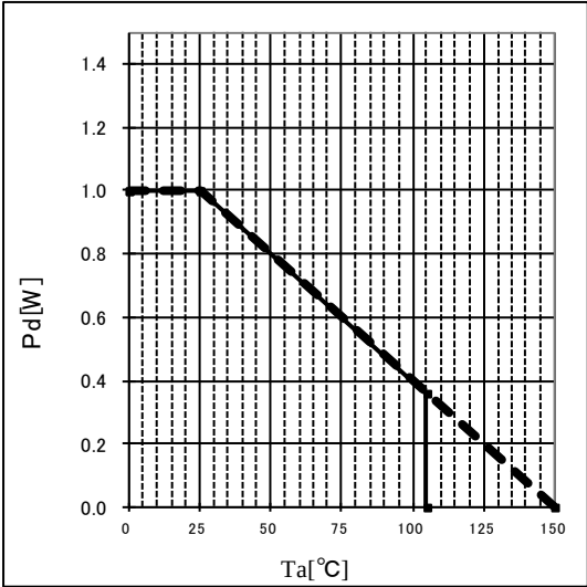
Figure 14. 熱軽減特性
