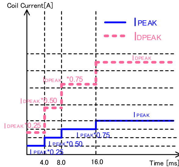
Figure 13. ソフトスタート動作
