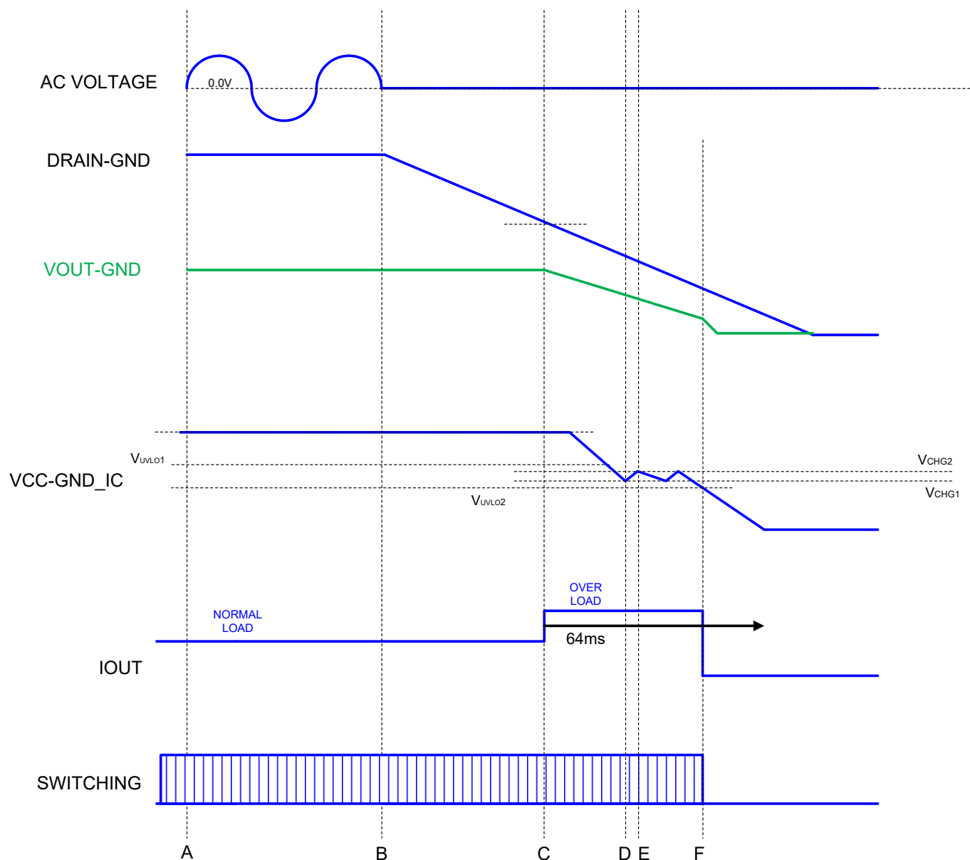
Figure 4. 停止シーケンス タイムチャート
