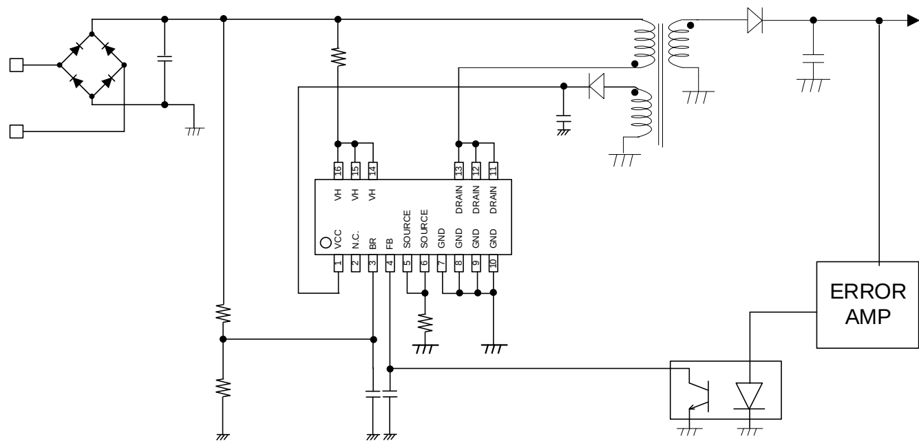
端子配置図
