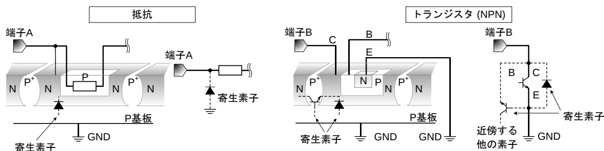
Figure 40. IC 構造例
