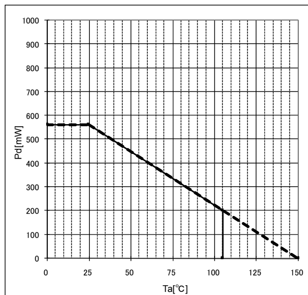
Figure 18. 熱軽減特性
