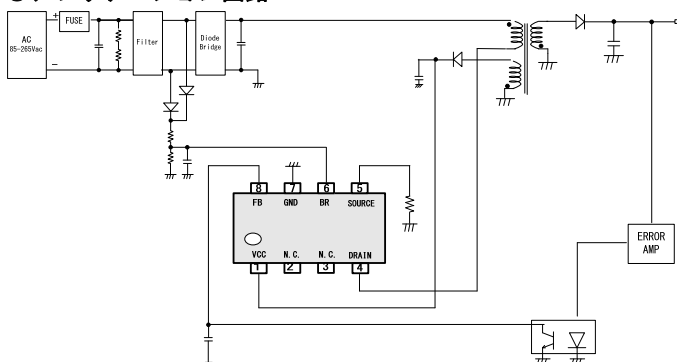
Figure 1. アプリケーション回路
