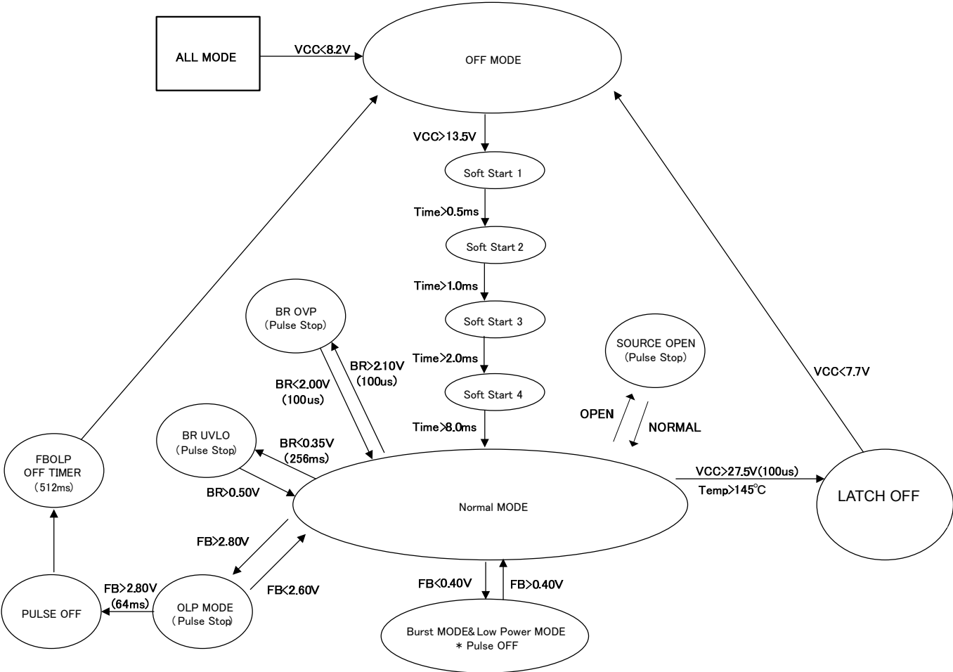
Figure 17. 状態遷移図
