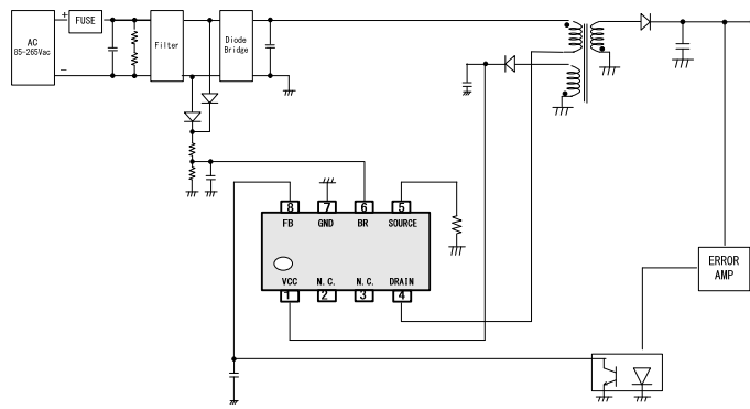
Figure 16(a). AC 電圧モニタ設定
