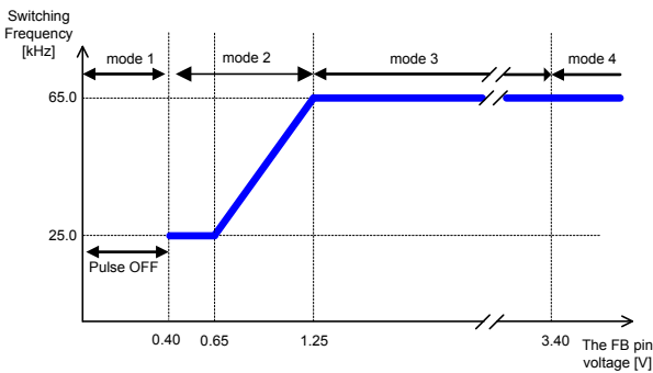
Figure 5A. スイッチング周波数 vs FB 端子電圧 (BM2P061HK-LBZ)
