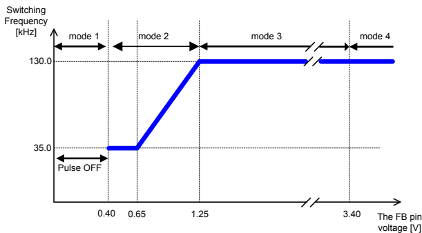
Figure 5C. スイッチング周波数 vs FB 端子電圧 (BM2P131HK-LBZ)
