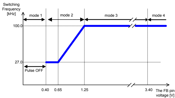
Figure 5B. スイッチング周波数 vs FB 端子電圧 (BM2P101HK-LBZ)
