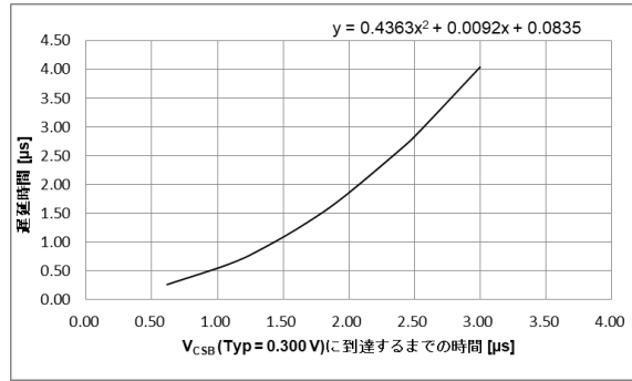
Figure 6B. 遅延時間 vs V_{CSB} (Typ = 0.300 V) に到達するまでの時間(BM2P101HK-LBZ)
