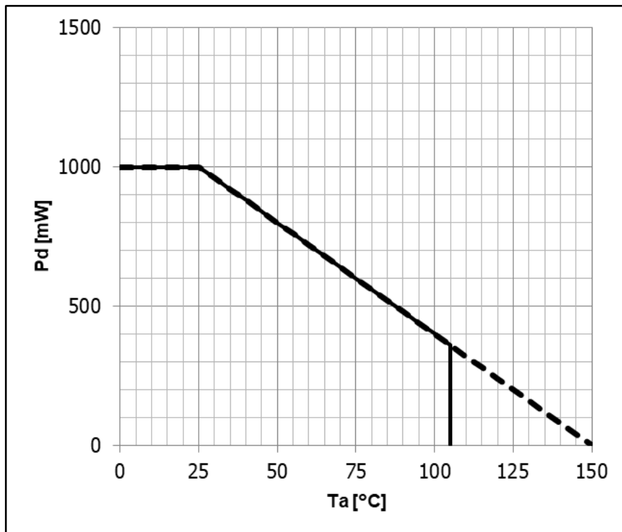
Figure 13. 熱軽減特性
