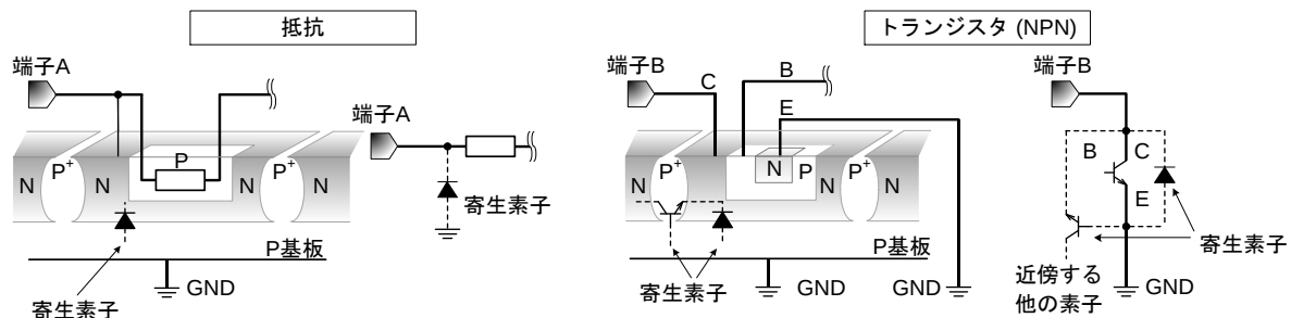
Figure 48. IC 構造例
