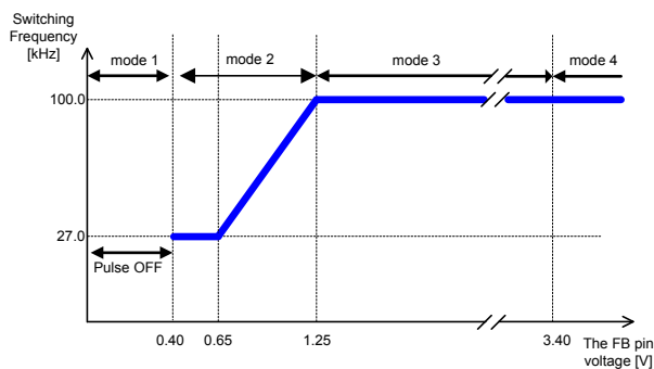
Figure 5B. スイッチング周波数 vs FB 端子電圧 (BM2P103HK-LBZ)
