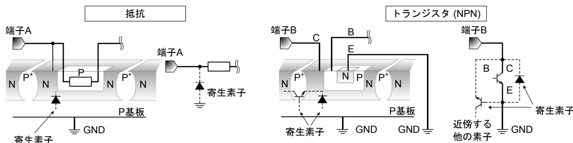
Figure 14. IC 構造例
