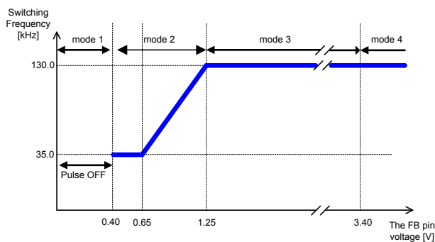
Figure 5C. スイッチング周波数 vs FB 端子電圧 (BM2P133HK-LBZ)
