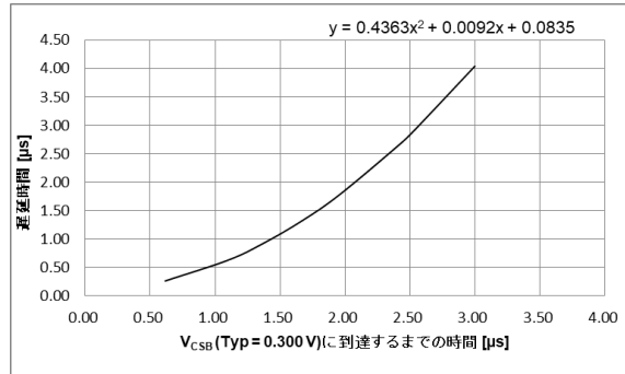
Figure 6B. 遅延時間 vs V_{CSB} (Typ = 0.300 V) に到達するまでの時間(BM2P103HK-LBZ)
