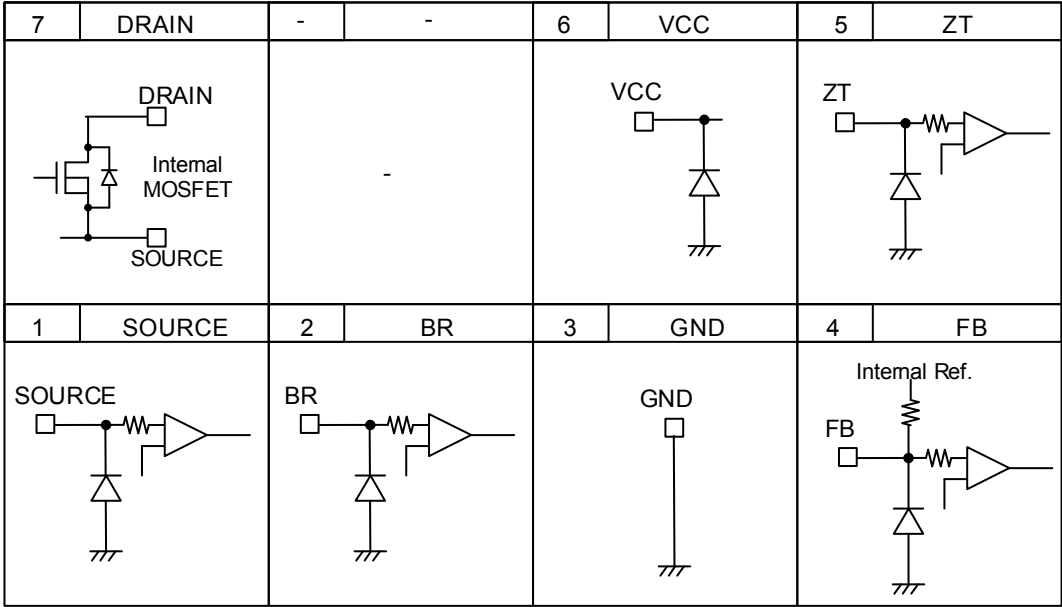
入出力等価回路図
