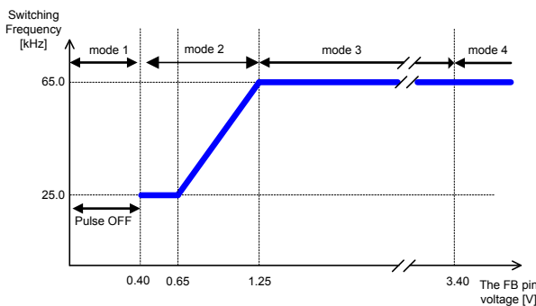
Figure 5A. スイッチング周波数 vs FB 端子電圧 (BM2P063HK-LBZ)
