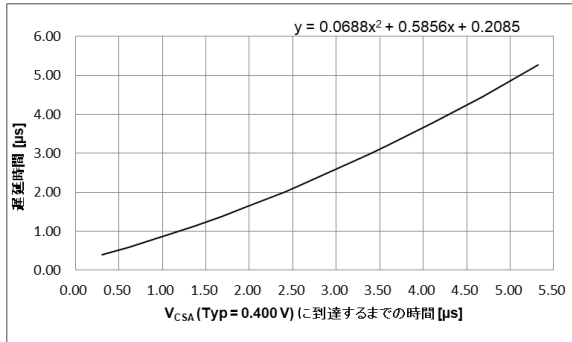
Figure 6A. 遅延時間 vs V_{CSA} (Typ = 0.400 V) に到達するまでの時間(BM2P063HK-LBZ)
