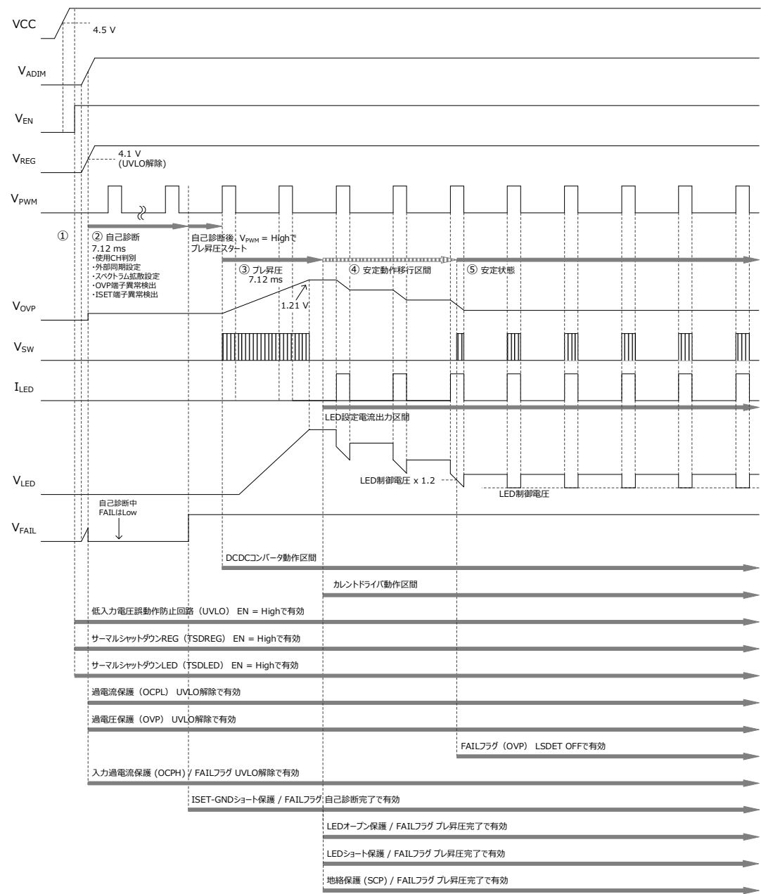
Figure 27. 起動時のタイミングチャートと各保護機能の有効区間 (V ADIM = V REG 時)
