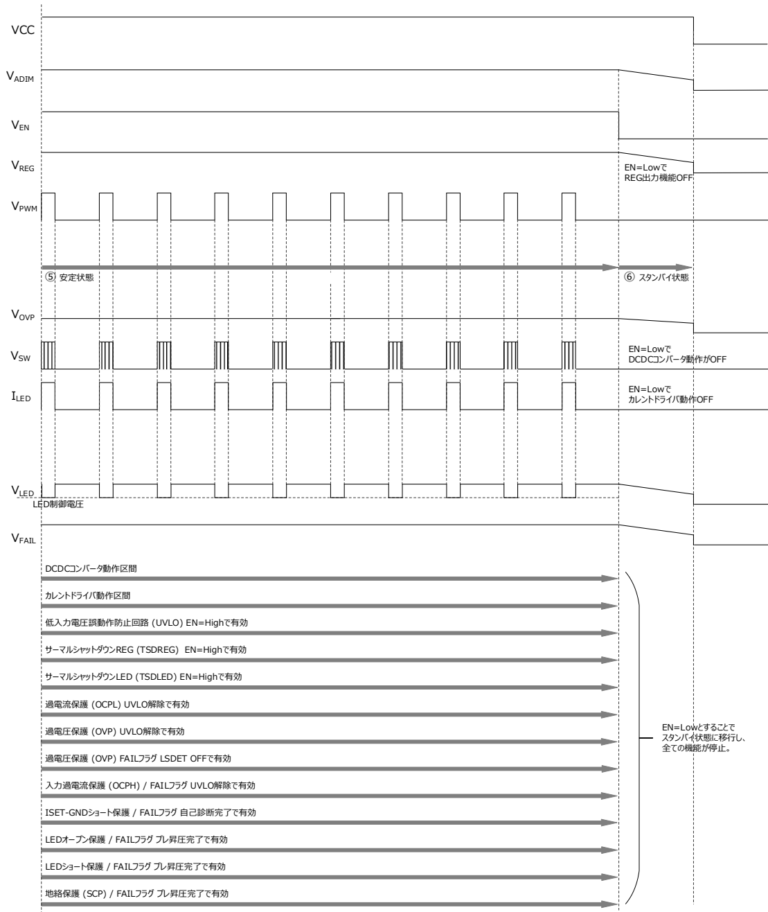
Figure 28. 停止時のタイミングチャートと各保護機能の有効区間 (VADIM = VREG 時)
