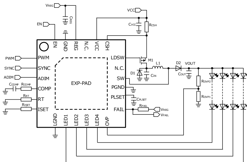
Figure 1. 昇圧アプリケーション回路図
