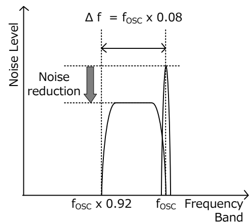
Figure 23. スペクトラム拡散機能
