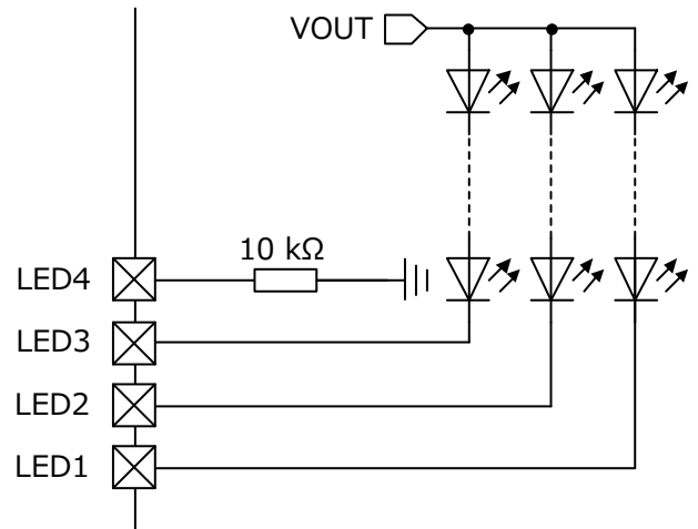
Figure 13. LED4 を未使用設定する場合
