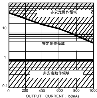
Fig.33 ESR - Io 特性 (BAxxCC0, 22µF)
