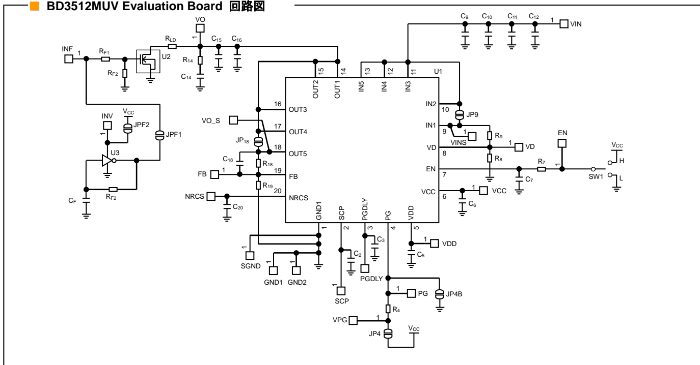
■ BD3512MUV Evaluation Board 回路図
