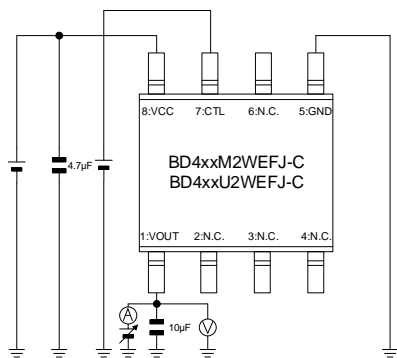
Figure 10、28 の測定回路図
