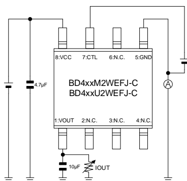
Figure 13、31 の測定回路図
