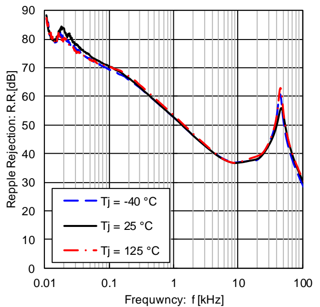
Figure 30. リップルリジェクション ( e_{in}=1\text{Vrms} 、 I_{OUT}=100\text{mA} )
