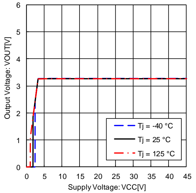
Figure 6. 出力電圧電源特性 (IOUT=0mA)
