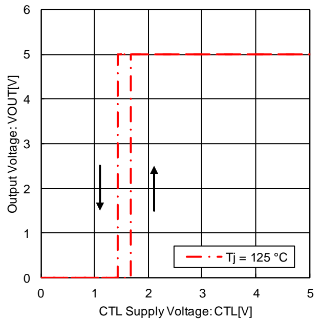
Figure 38. CTL 端子 ON / OFF モード電圧 (Tj=125°C)
