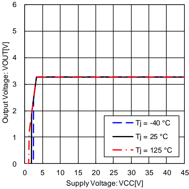
Figure 9. 出力電圧電源特性 ( I_{OUT}=10\text{mA} )
