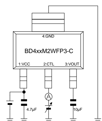
Figure 22、40 の測定回路図
