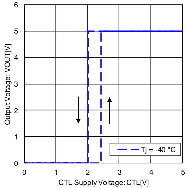
Figure 36. CTL 端子 ON / OFF モード電圧 (Tj=-40°C)
