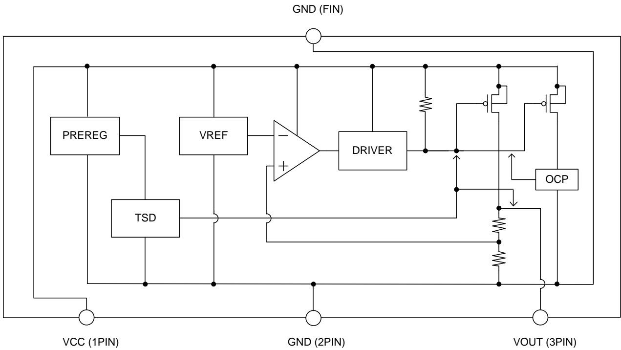
Figure 4. ブロック図
