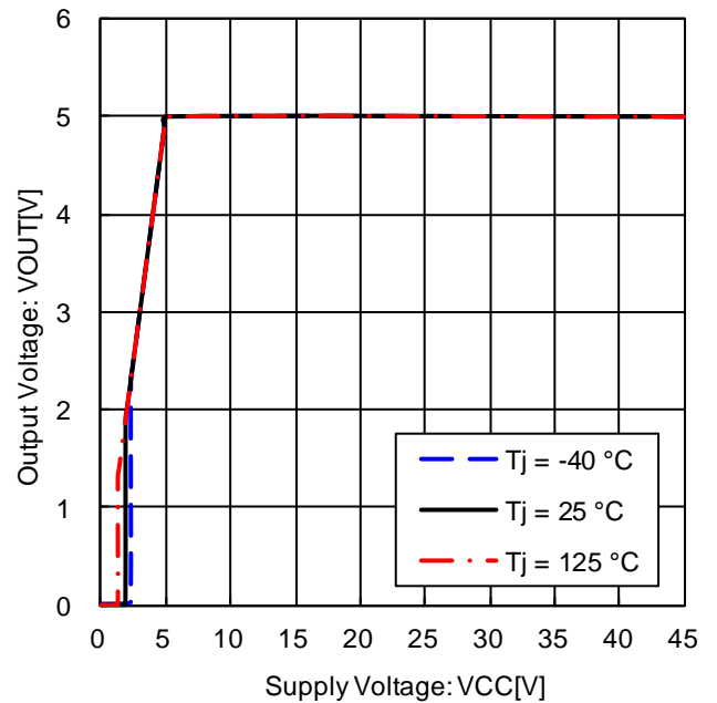
Figure 24. 出力電圧電源特性 (IOUT=0mA)
