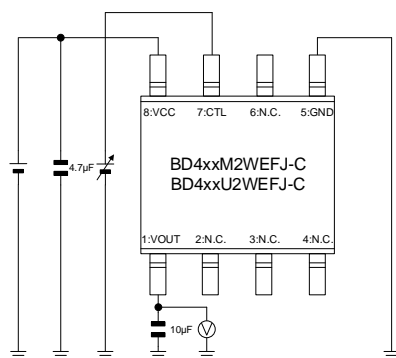
Figure 18、19、20、 Figure 36、37、38 の測定回路図
