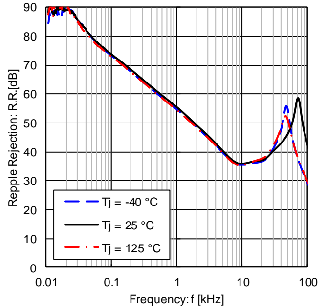
Figure 12. リプルリジェクション ( e_{in}=1\text{V}_{rms} 、 I_{OUT}=100\text{mA} )
