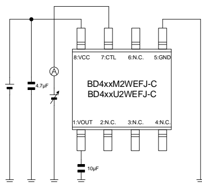
Figure 22、40 の測定回路図
