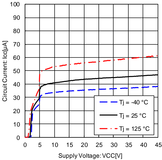
Figure 23. 回路電流
