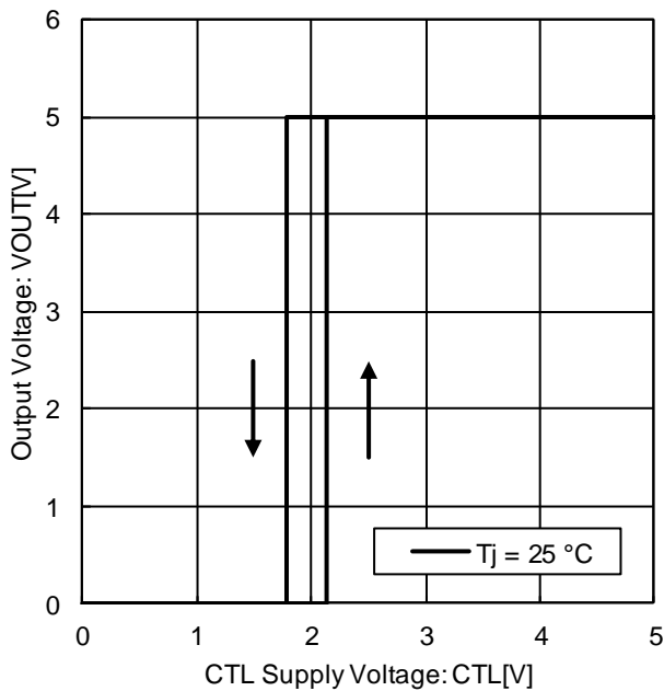
Figure 37. CTL 端子 ON / OFF モード電圧 (Tj=25°C)
