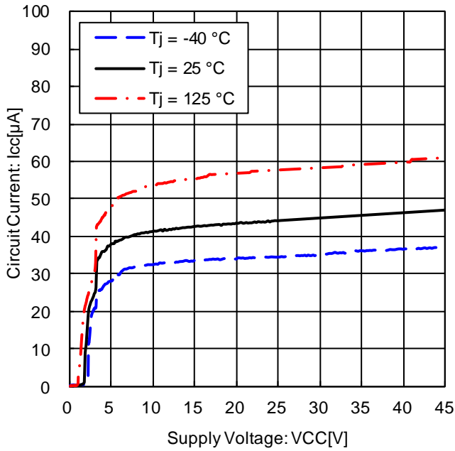
Figure 5. 回路電流
