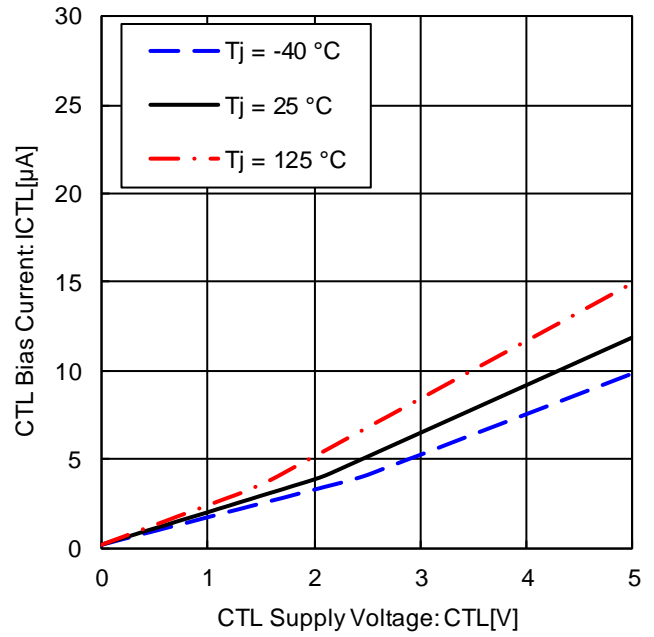
Figure 22. CTL バイアス電流 vs. CTL 電圧
