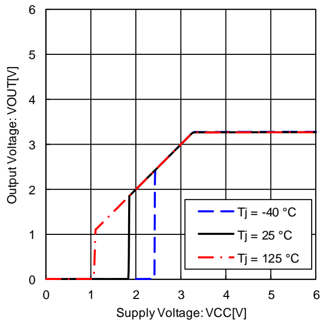
Figure 8. 出力電圧電源特性 (IOUT=0mA) ※電源電圧が低いとき
