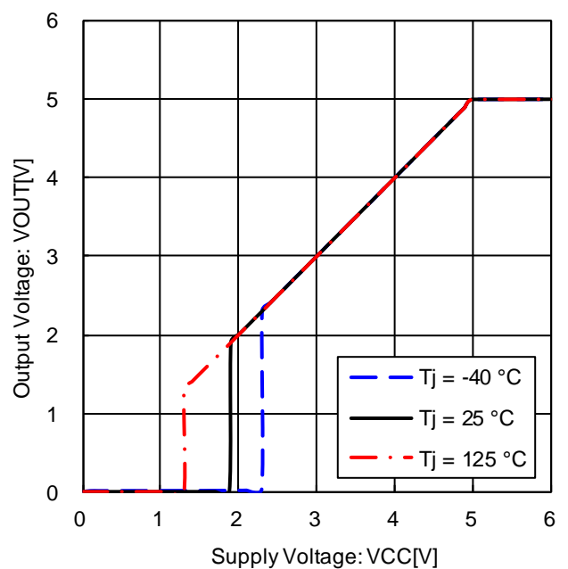
Figure 26. 出力電圧電源特性 (IOUT=0mA) ※電源電圧が低いとき
