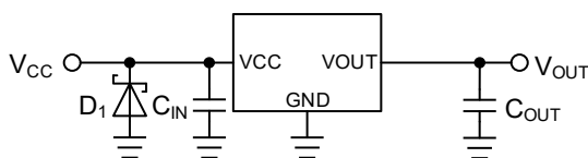
Figure 44. 入力に-0.3 V を超える負サージが印加される場合
