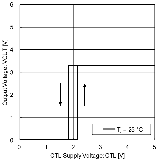
Figure 18. CTL 端子 ON / OFF モード電圧 (Tj = 25 °C)
