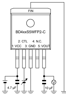
Figure 17、18、19、 Figure 35、36、37 の測定回路図
