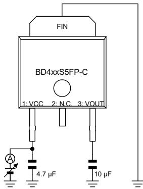
Figure 4、6、15、 Figure 22、24、33 の測定回路図
