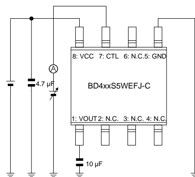
Figure 21、39 の測定回路図
