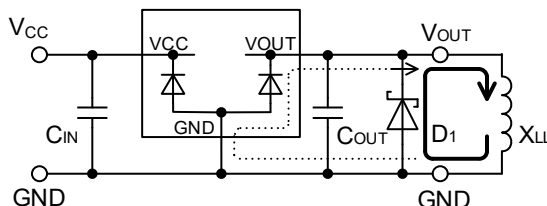
Figure 52. 誘導性負荷の電流経路 (出力 OFF 時)
