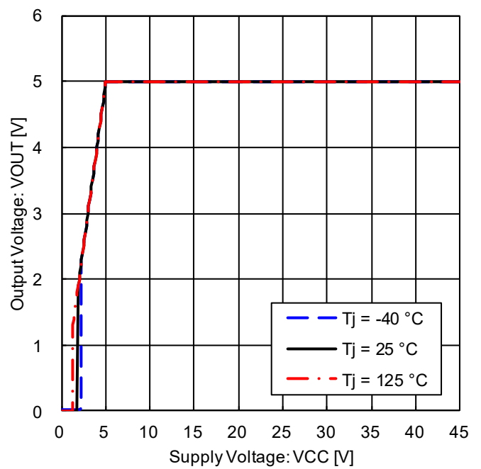
Figure 23. 出力電圧電源特性 ( I_{OUT} = 0\text{ mA} )
