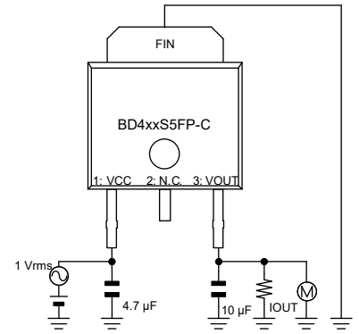
Figure 11、29 の測定回路図
