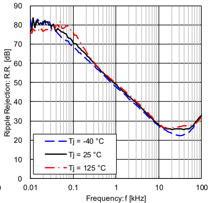
Figure 11. リップルリジェクション ( e_{in} = 1\text{ V}_{rms} 、 I_{OUT} = 100\text{ mA} )
