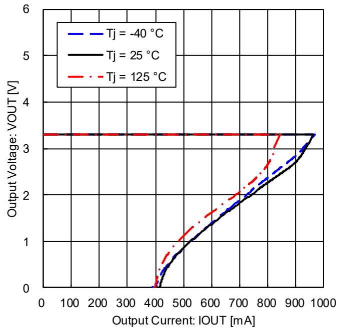
Figure 9. 出力電圧負荷特性 (過電流保護特性)
