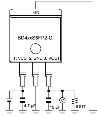
Figure 8、26 の測定回路図
