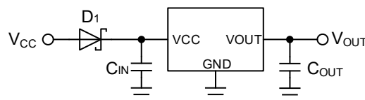
Figure 49. 逆接続対策 1
