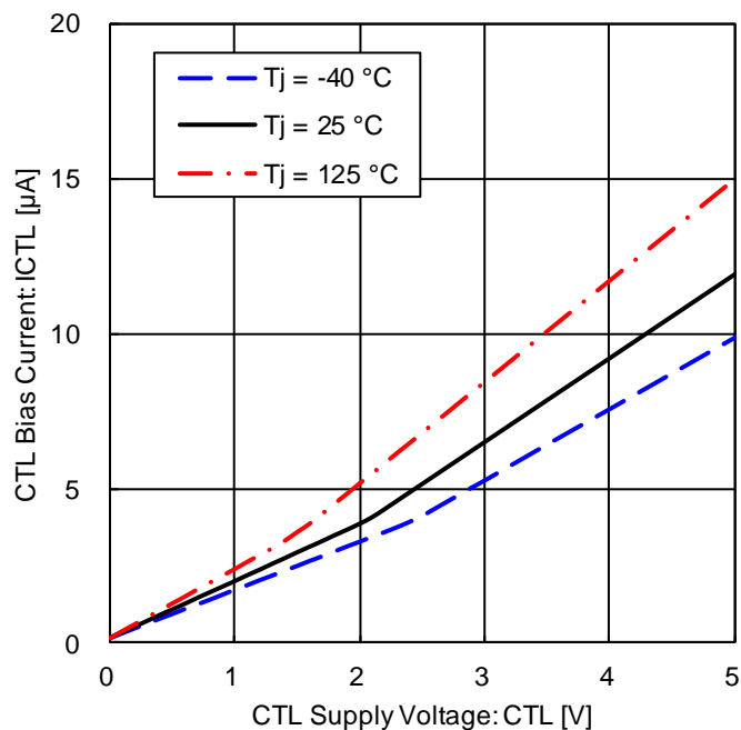
Figure 39. CTL バイアス電流 vs CTL 電圧
