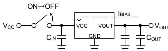
Figure 47. 入力をオープンにした場合
