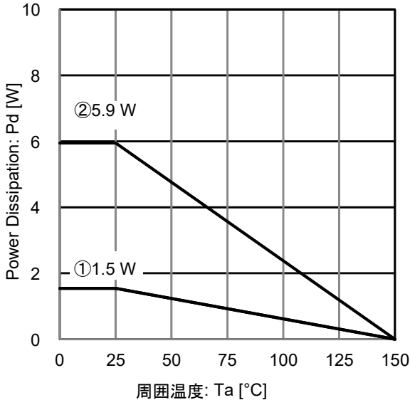
Figure 54. 熱低減曲線グラフ (TO263-3 / TO263-5)
