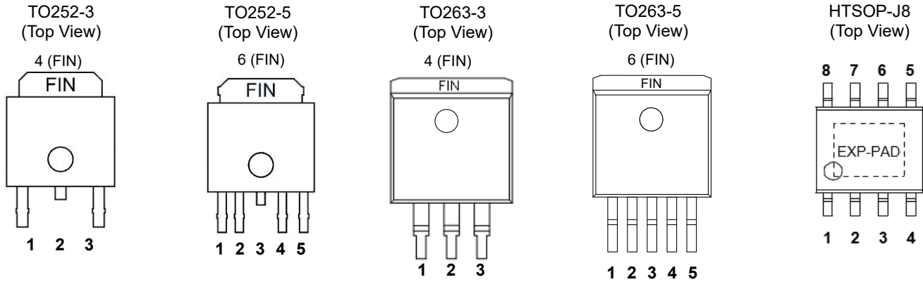
Figure 3. 端子配置図
