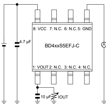
Figure 12、30 の測定回路図
