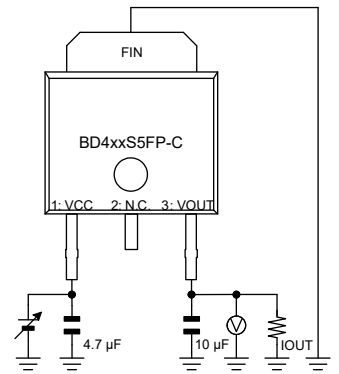
Figure 8、26 の測定回路図
