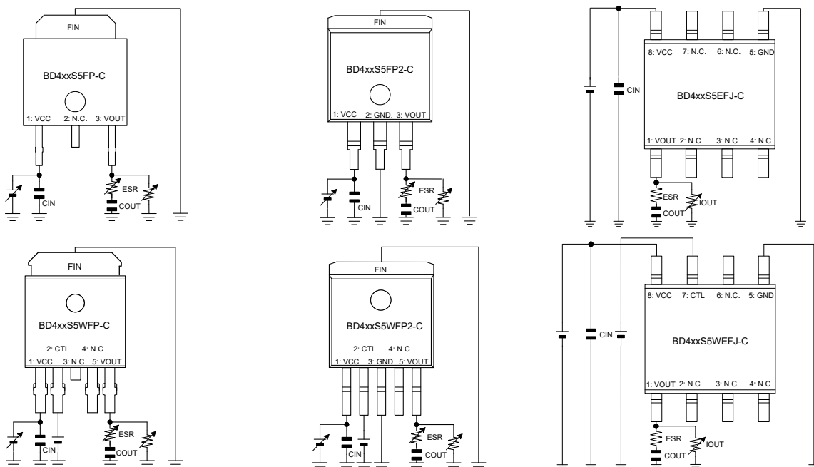
Figure 42. 出力端子接続コンデンサ特性 測定回路図
