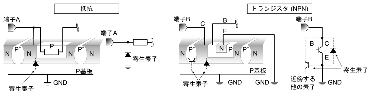
Figure 57. モノリシック IC 構造例
