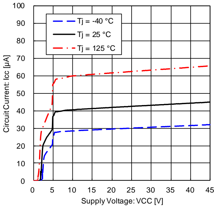
Figure 22. 回路電流
