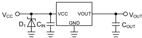
Figure 43. 入力に 45 V を超えるサージが印加される場合
