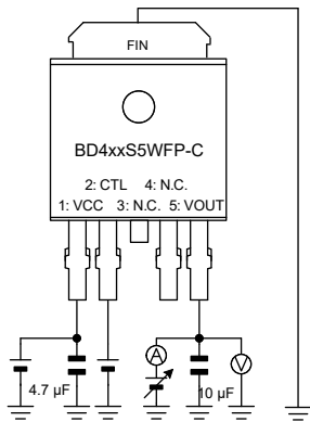
Figure 9、27 の測定回路図
