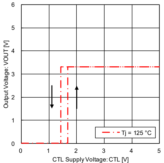
Figure 19. CTL 端子 ON / OFF モード電圧 (Tj = 125 °C)
