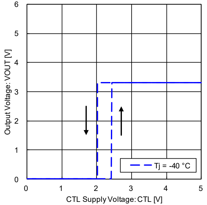
Figure 17. CTL 端子 ON / OFF モード電圧 (Tj = -40 °C)
