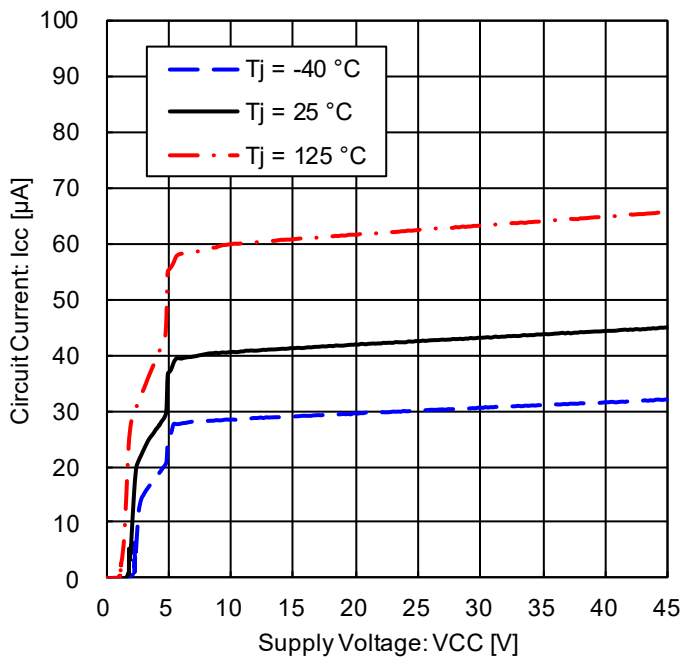
Figure 22. 回路電流
