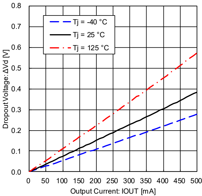
Figure 10. 最小入出力電圧差 ( V_{CC} = 3.135\text{ V} )
