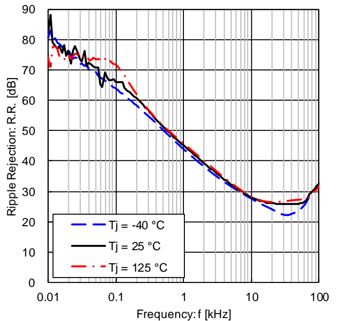
Figure 29. リップルリジェクション ( e_{in} = 1\text{ V}_{rms} 、 I_{OUT} = 100\text{ mA} )
