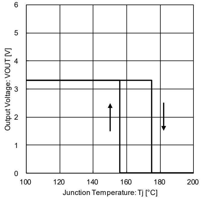
Figure 13. 温度保護回路特性
