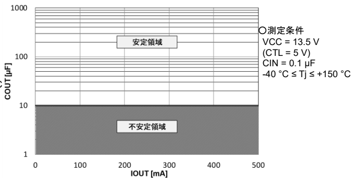
Figure 41. COUT (Typ) vs 出力電流 (IOUT)
