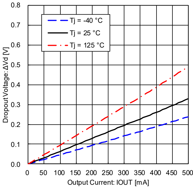
Figure 28. 最小入出力電圧差 ( V_{CC} = 4.75\text{ V} )
