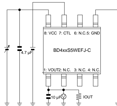
Figure 8、26 の測定回路図
