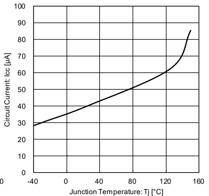
Figure 33. 回路電流温度特性
