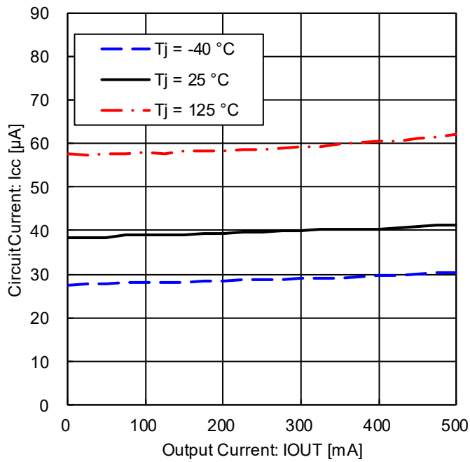
Figure 12. 負荷別回路電流
