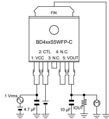
Figure 11、29 の測定回路図
