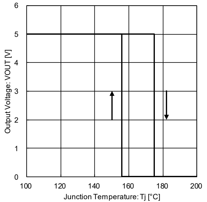
Figure 31. 温度保護回路特性
