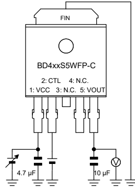
Figure 5、7、13、14、 Figure 23、25、31、32 の測定回路図
