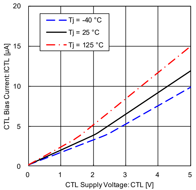
Figure 39. CTL バイアス電流 vs CTL 電圧
