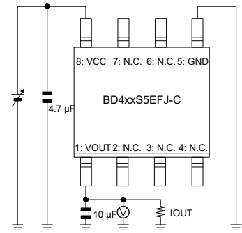
Figure 8、26 の測定回路図
