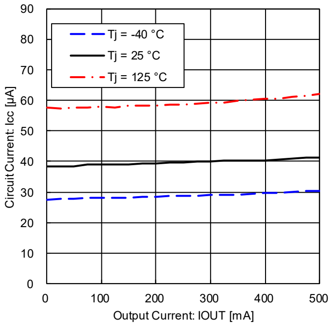
Figure 30. 負荷別回路電流
