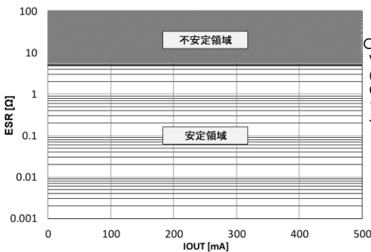
Figure 40. ESR vs 出力電流 (IOUT)
