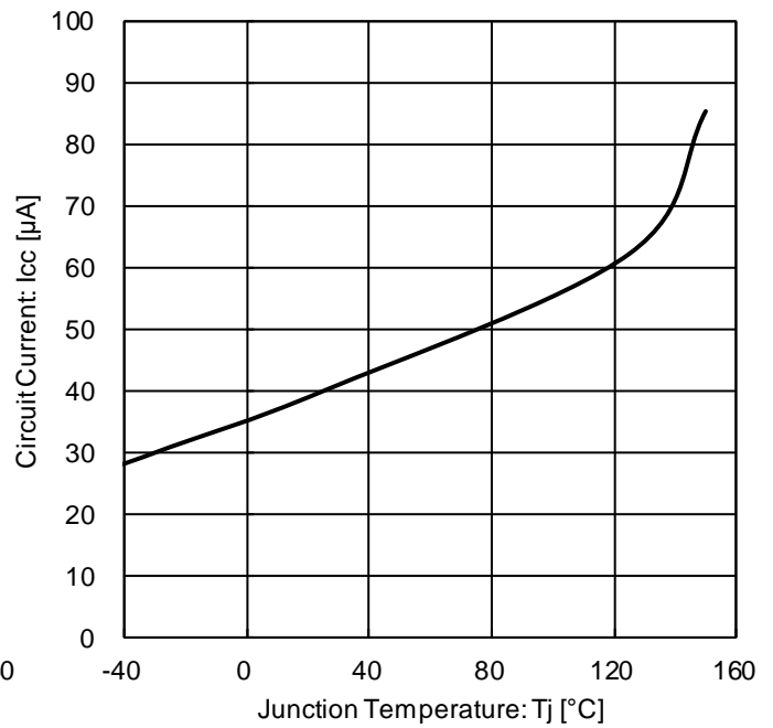
Figure 15. 回路電流温度特性
