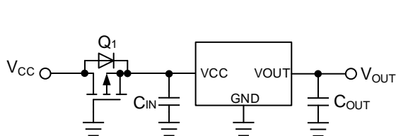
Figure 50. 逆接続対策 2
