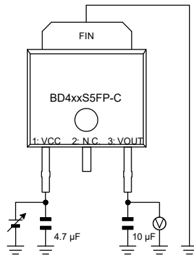
Figure 5、7、13、14、 Figure 23、25、31、32 の測定回路図
