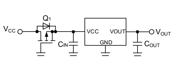
Figure 50. 逆接続対策 2
