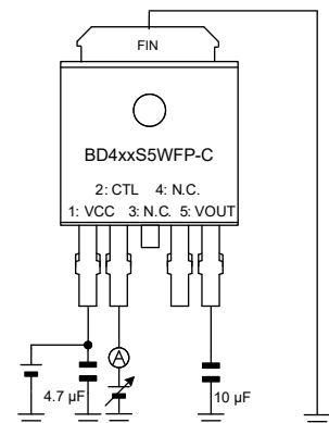
Figure 21、39 の測定回路図
