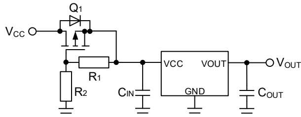
Figure 51. 逆接続対策 3
