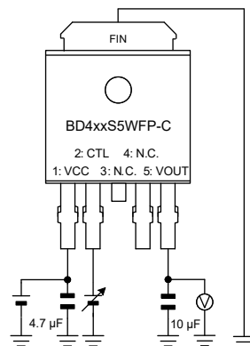
Figure 17、18、19、 Figure 35、36、37 の測定回路図
