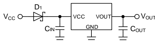
Figure 49. 逆接続対策 1
