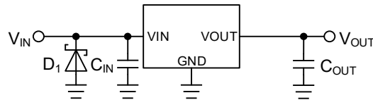
Figure 74. 入力に-0.3 V を超える負サージが印加される場合
