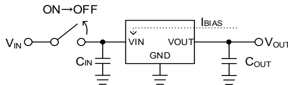
Figure 77. 入力をオープンにした場合
