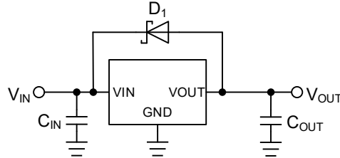
Figure 76. 逆電流バイパスダイオード
