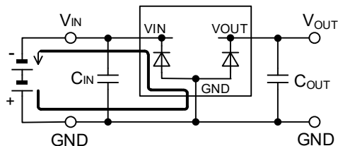
Figure 78. 入力を逆接続したときの電流経路
