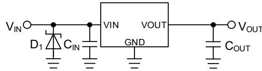
Figure 73. 入力に絶対最大定格を超えるサージが印加される場合
