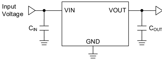
出力シャットダウン機能無し
