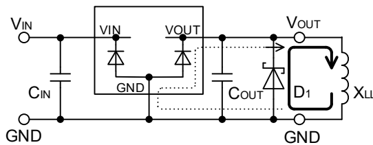
Figure 82. 誘導性負荷の電流経路 (出力 OFF 時)
