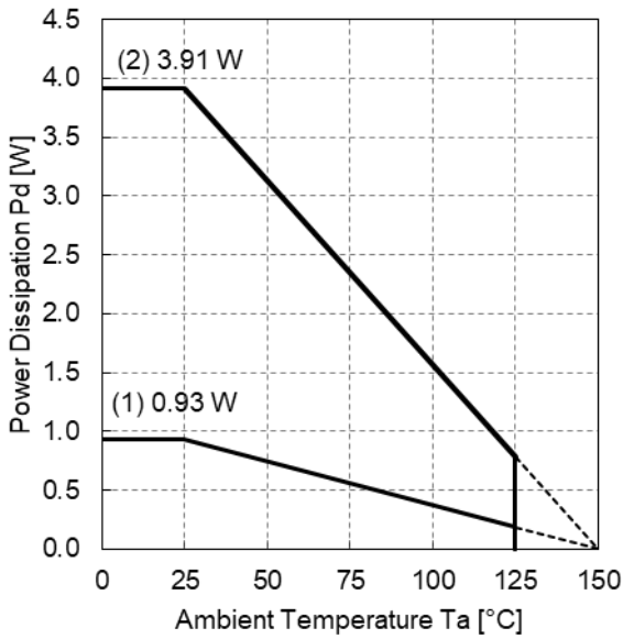
Figure 83. 許容損失グラフ (HTSOP-J8)
