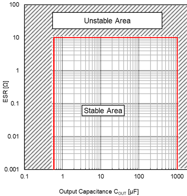
Figure 72. 出力端子コンデンサ容量値、ESR 安定動作領域 ( V_{IN} = 3\text{ V} \sim 42\text{ V} 、 V_{OUT} = 1.5\text{ V} (Note 1) 、 -40\text{ }^{\circ}\text{C} \leq T_j \leq +150\text{ }^{\circ}\text{C} 、 I_{OUT} = 0\text{ mA} \sim 500\text{ mA} ) (Note 1) レギュレータの制御ループの安定性理論から最も厳しい条件
