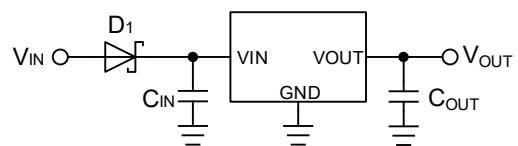
Figure 79. 逆接続対策 1
