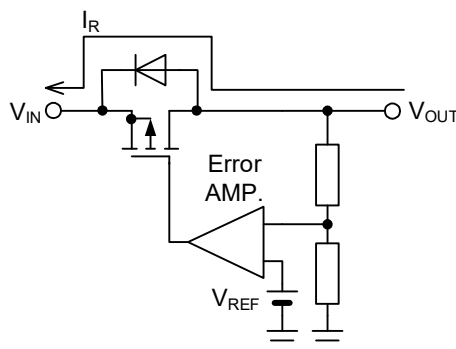
Figure 75. MOS 型リニアレギュレータの逆電流経路
