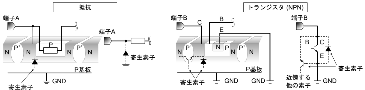
Figure 84. モノリシック IC 構造例
