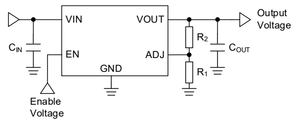
出力シャットダウン機能有り
