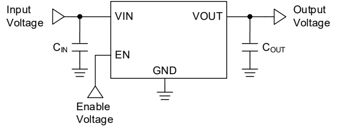
出力シャットダウン機能有り
