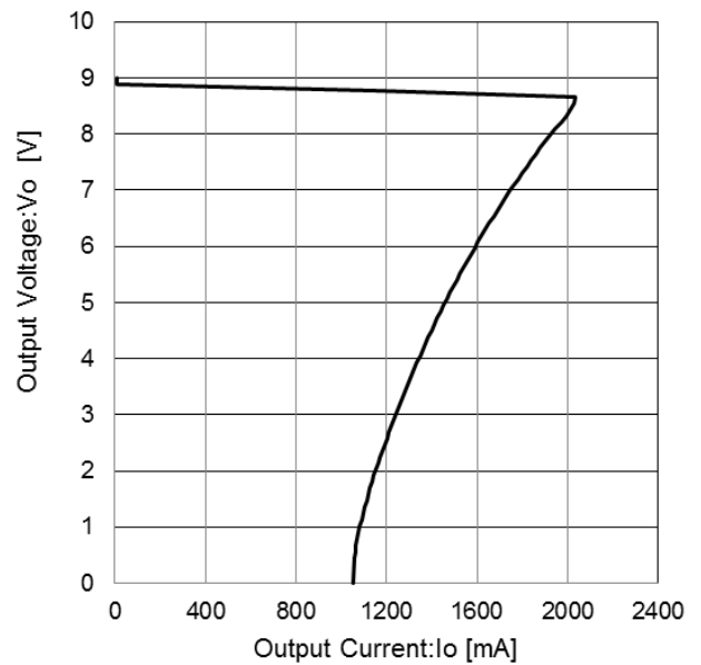
Figure 16. 負荷安定度
