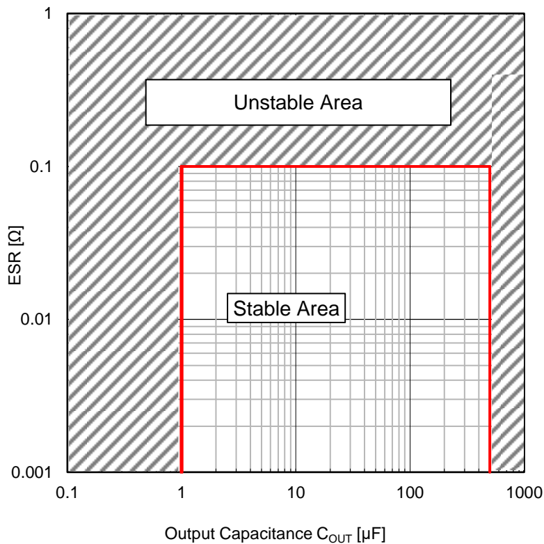
Figure 55. 出力端子コンデンサ容量値、ESR 安定動作領域 (V_{IN} = 4.5 \text{ V} \sim 42 \text{ V}, V_{OUT} = 1 \text{ V}^{(Note 1)}, -40 \text{ }^\circ\text{C} \leq T_j \leq +150 \text{ }^\circ\text{C}, I_{OUT} = 0 \text{ mA} \sim 500 \text{ mA}) (Note 1) レギュレータの制御ループの安定性理論から最も厳しい条件
