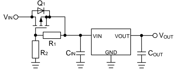
Figure 64. 逆接続対策 3
