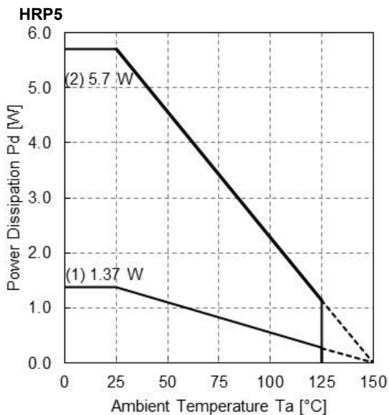
Figure 67. 許容損失グラフ (HRP5)
