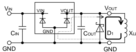
Figure 65. 誘導性負荷の電流経路 (出力 OFF 時)
