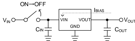
Figure 60. 入力をオープンにした場合
