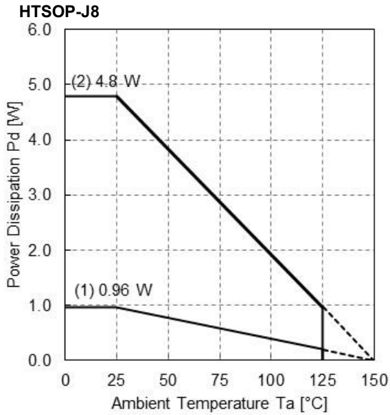
Figure 68. 許容損失グラフ (HTSOP-J8)
