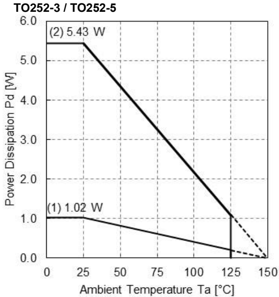
Figure 66. 許容損失グラフ (TO252-3 / TO252-5)
