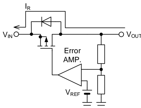
Figure 58. MOS 型リニアレギュレータの逆電流経路
