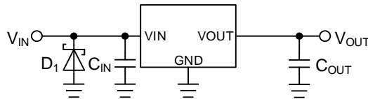
Figure 57. 入力に-0.3 V を超える負サージが印加される場合
