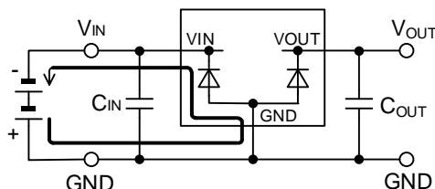
Figure 61. 入力を逆接続したときの電流経路
