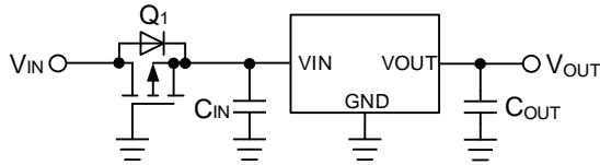
Figure 63. 逆接続対策 2
