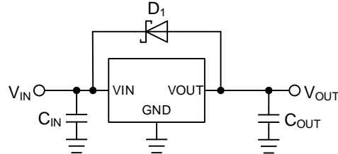
Figure 59. 逆電流バイパスダイオード
