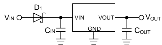
Figure 62. 逆接続対策 1
