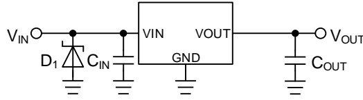
Figure 56. 入力に絶対最大定格を超えるサージが印加される場合
