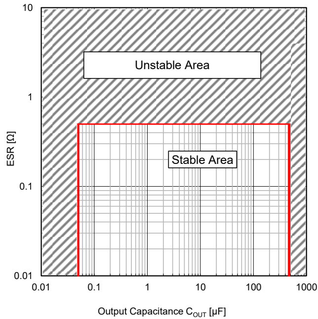
Figure 51. 出力端子コンデンサ容量値、ESR 安定動作領域 (-40 °C ≤ T j ≤ +150 °C、4.5 V ≤ V IN ≤ 42 V、V EN = 5 V、I OUT = 0 mA ~ 150 mA)
