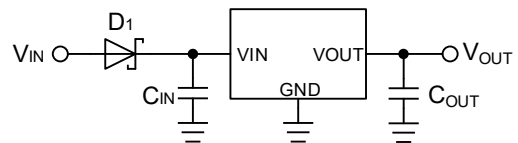
Figure 58. 逆接続対策 1
