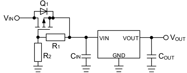
Figure 60. 逆接続対策 3
