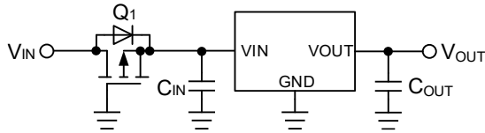
Figure 59. 逆接続対策 2
