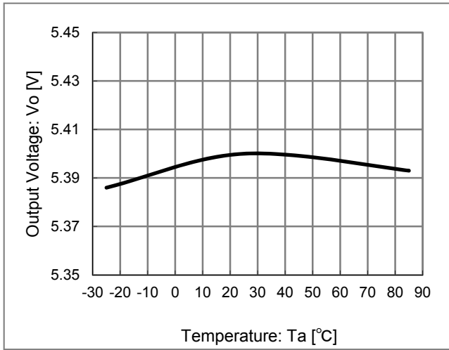
Figure 6. Ta - Vo (I o = 0mA)
