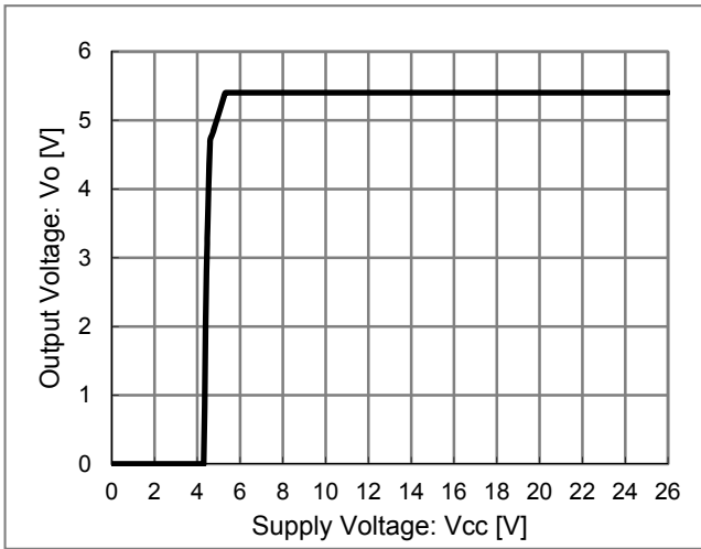
Figure 2. Vcc - Vo
