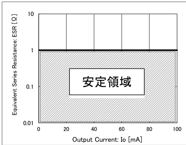
Figure 14 . ESR 安全動作領域
