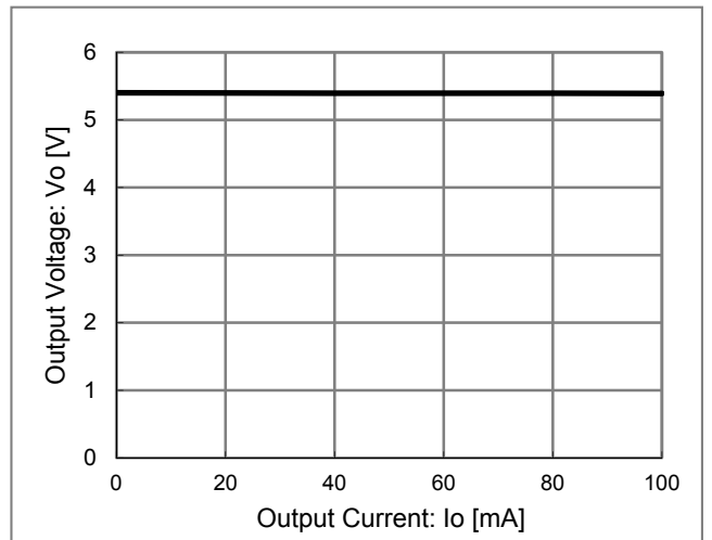
Figure 9. I o - Vo
