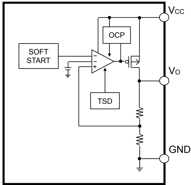
Figure 1. ブロック図
