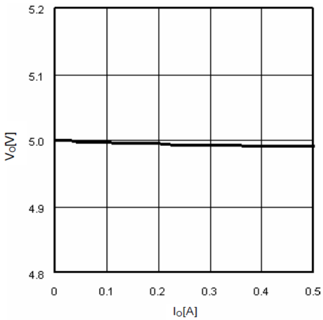
Fig. 25 I_o - V_o
