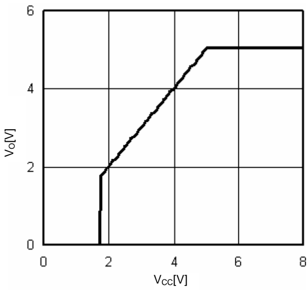
Fig.15 V_{cc}-V_o ( I_o=0mA )
