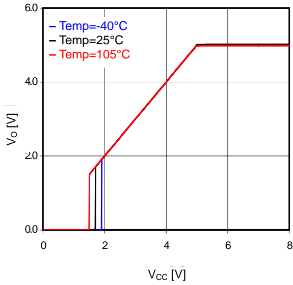
Fig. 27 V_{CC}-V_o ( I_o=0mA )
