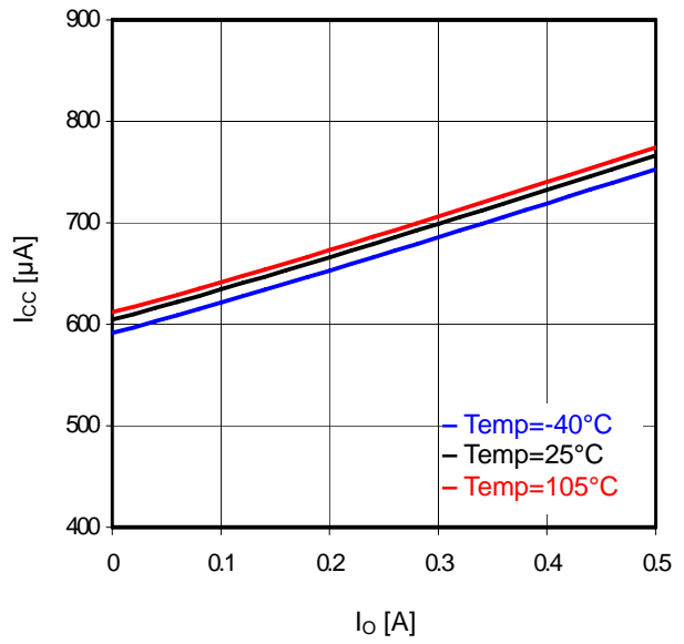
Fig. 30 I_o-I_{cc}
